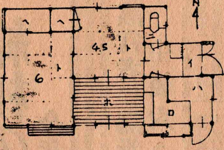
一種 B型 10.75坪 一戸建
