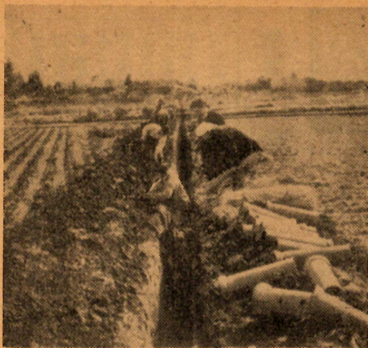
暗渠排水工事 只今暗渠排水工事を各地区で行つていますが、経営強化と生産力増強のためぜひ推進したいものです。(写真は上泉町内の暗渠工事)(農政部)
