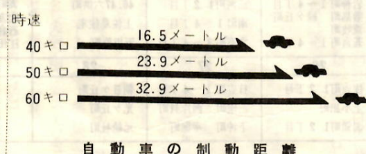
自動車の制動距離
