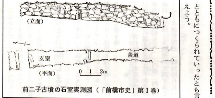
前二子古墳の石室実測図(「前橋市史」第1巻)
