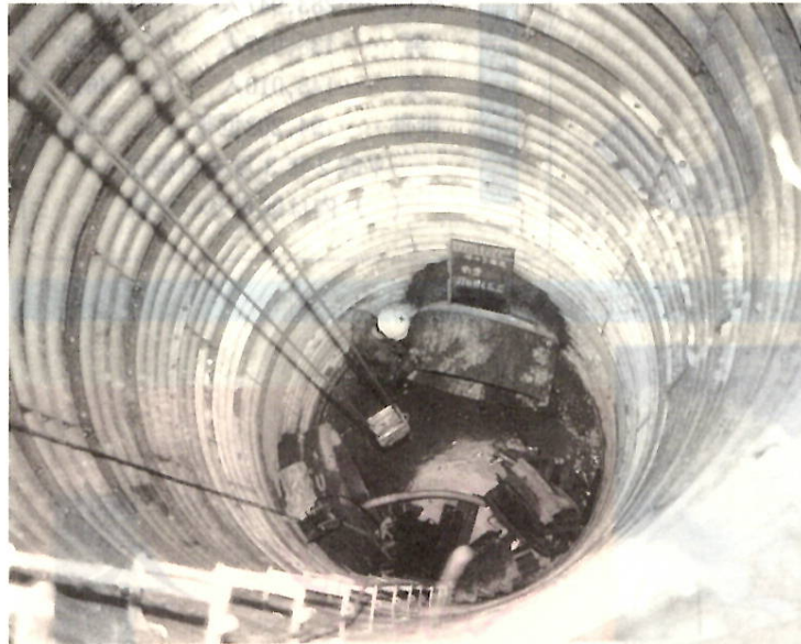
下水道工事は地下3mから10mを掘って進められます
