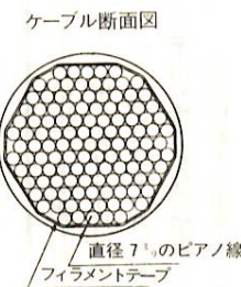
ケーブル断面図
