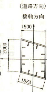
タワー断面図
