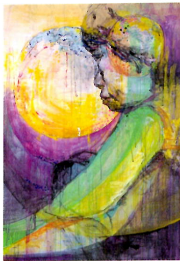
7月5日・月食(アクリル画)
