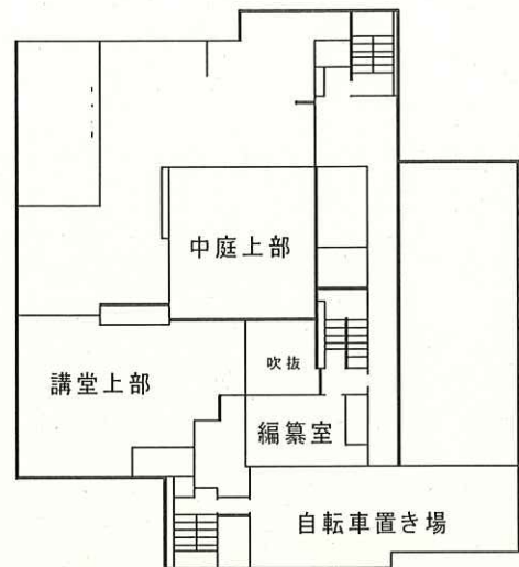
中地階
