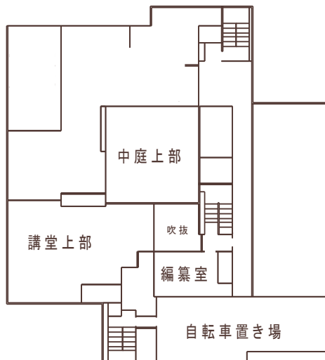
中地階
