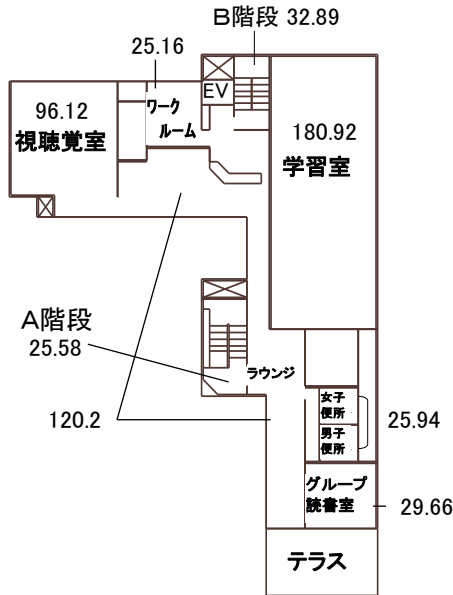
中地階(地下1階)平面図 【557.16m 2 】
