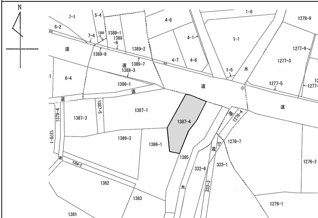
公図（縮尺1：1000）
