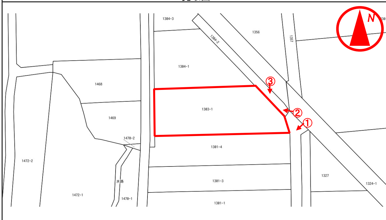
見取図
