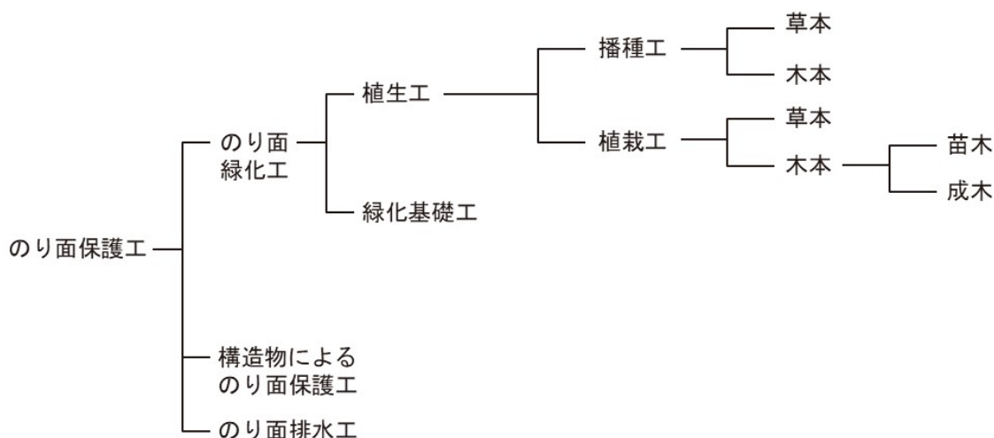
図 3-37 法面保護工の分類
