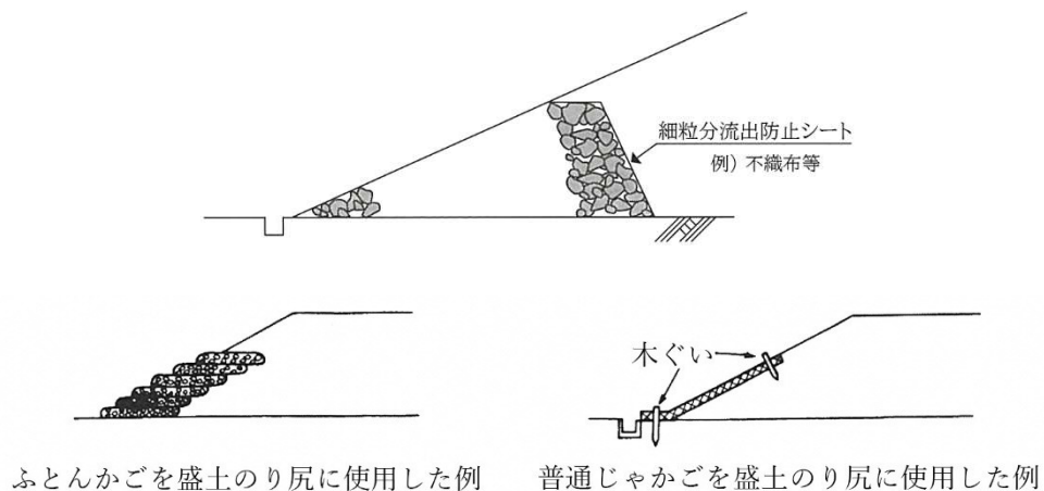
図 3-53 法尻工の例
