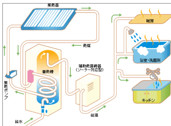
太陽熱利用温水器 (強制循環型)
