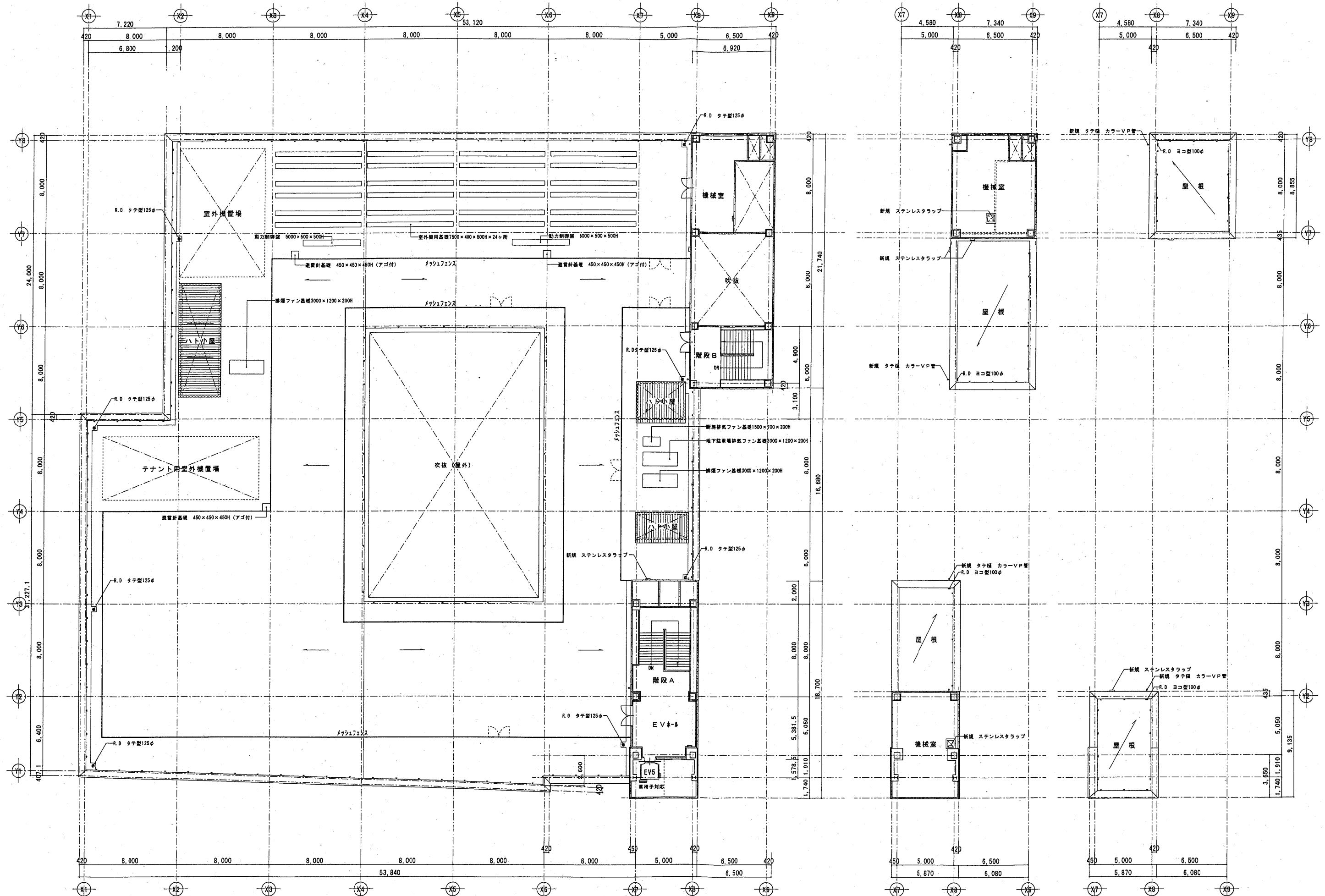
屋上一塔屋階平面図 1:300
