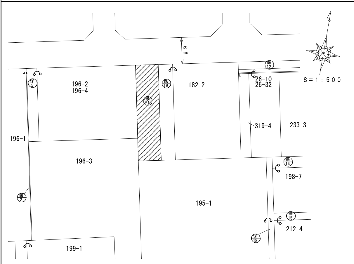
仮換地図
