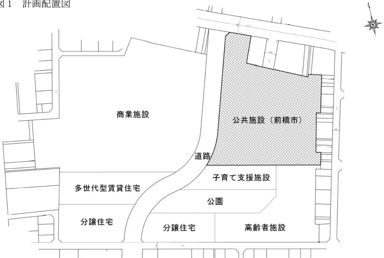
図 1 計画配置図
