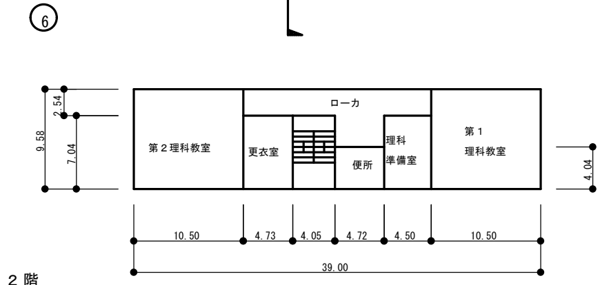
2階
