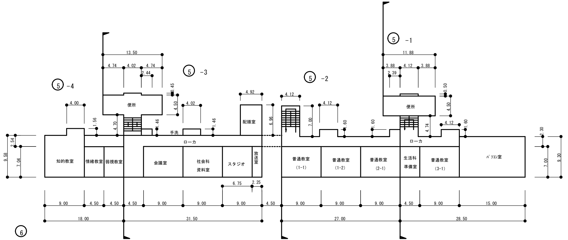
2階平面図
