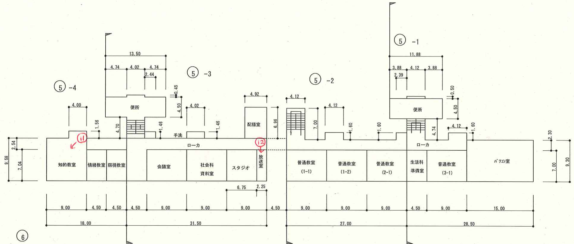
2階平面図
