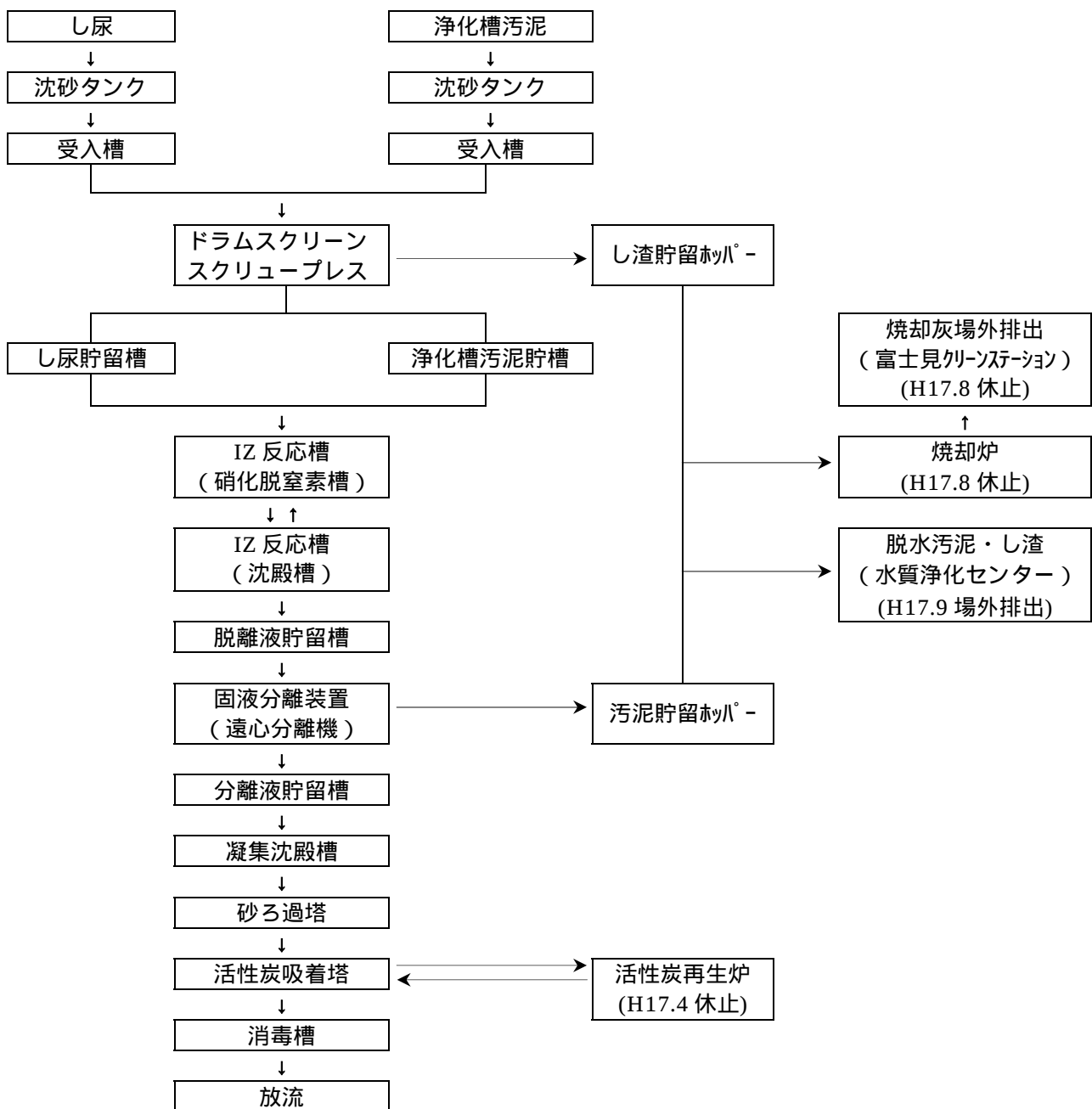
大胡衛生センターし尿処理施設フローシート
