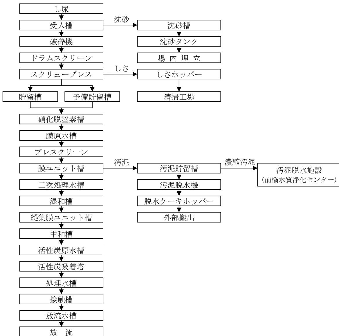
《し尿処理施設フローシート》
