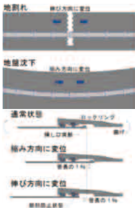
《耐震管のイメージ図》
