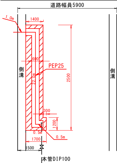
掘さく平面図
