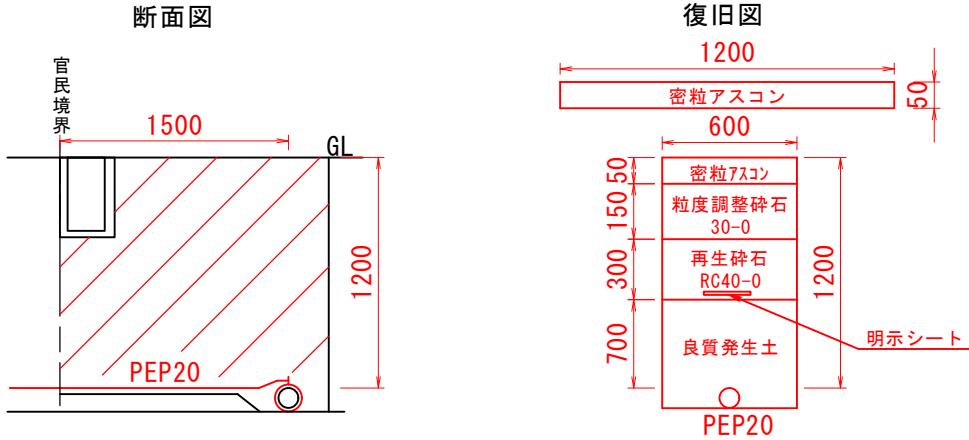
掘さく断面図及び復旧図
