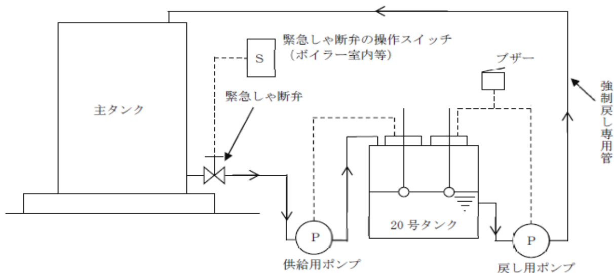
第3 -20 図 強制戻し専用管及び緊急しや断弁を設置する例
