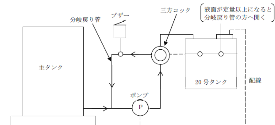
第 3 -16 図 分岐戻り管を設置する例
