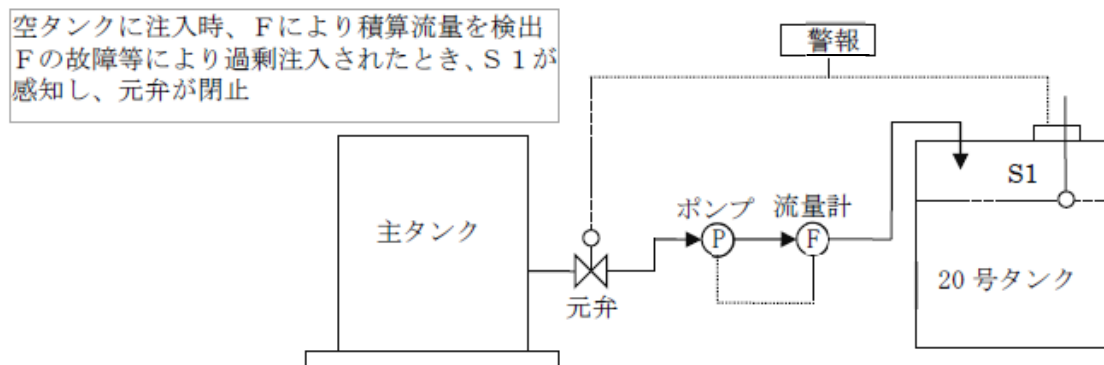
第3-14 図 流量計で注入量を計量し危険物注入用ポンプを停止させる設備と液面感知センサーで元弁を閉止する設備を設置する例
