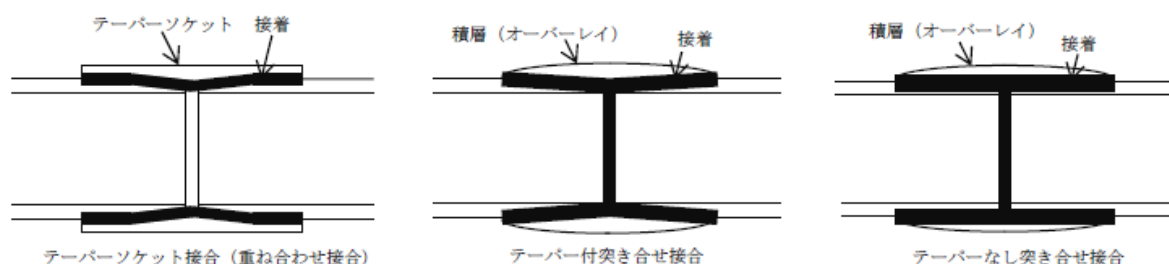
第3-23図 FRP配管の接着接合例
