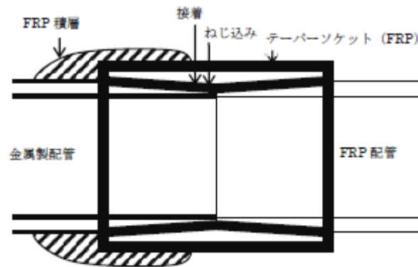
第3-24 図 トランジション継手の接着接合例
