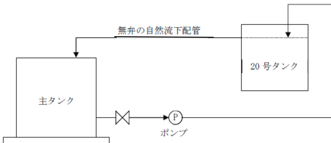
第 3－9 図 自然流下配管を設置する例
