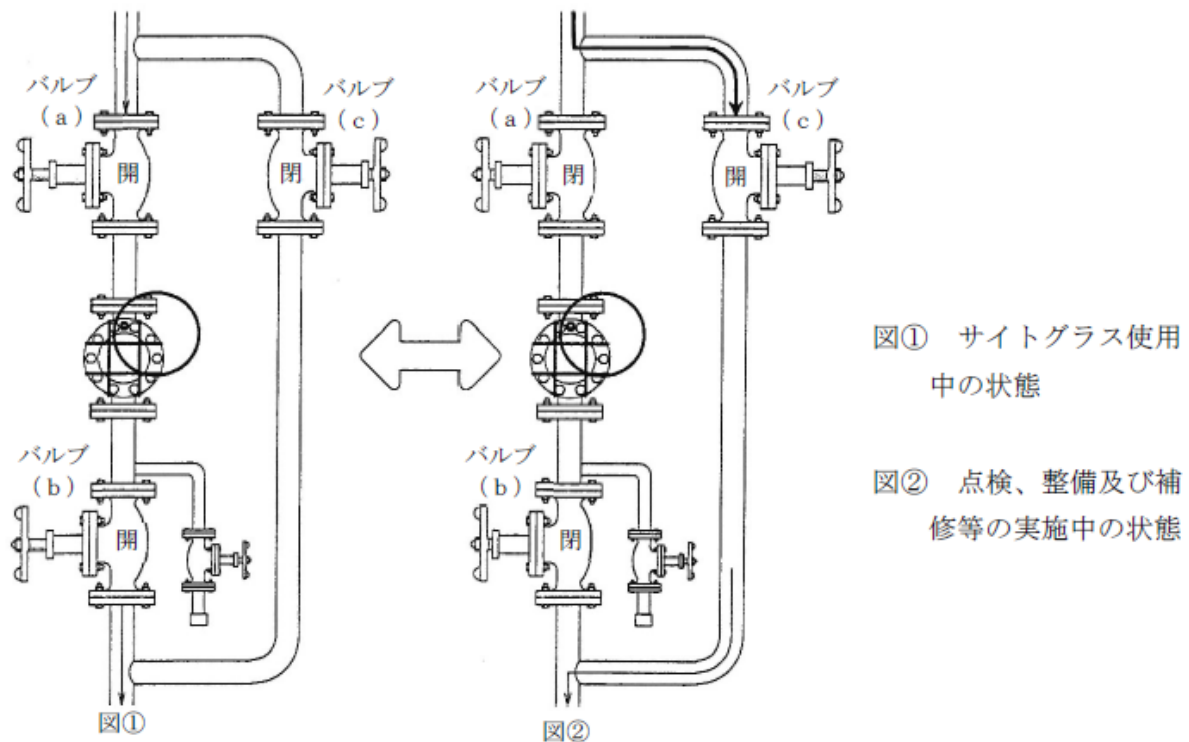
第3 -31図 サイトグラスを設けた配管の点検、整備及び補修等の操作方法 (第3 -31図 の場合の操作方法)
