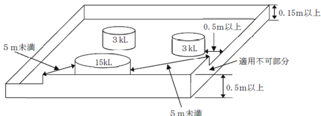
第3-15図 一部特例措置を適用できない20号防油堤の例
