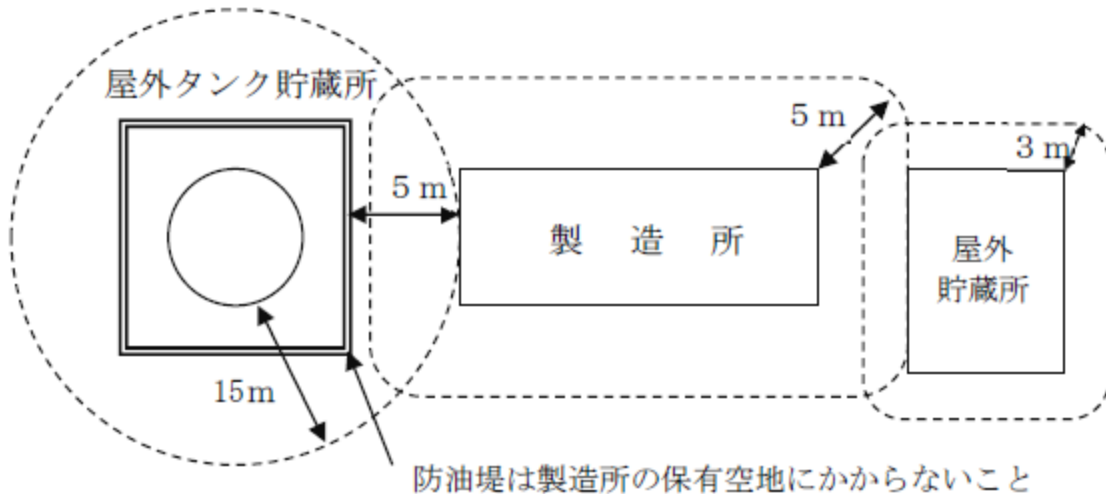
第3-1図 保有空地の例
