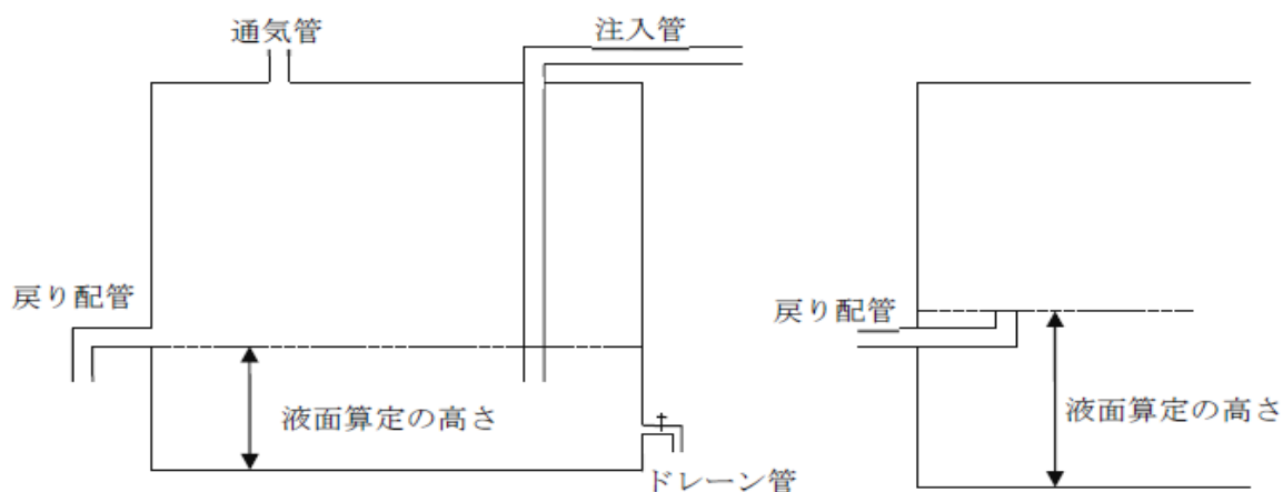
第3-6図 戻り配管を設けた20号タンクの液面算定
