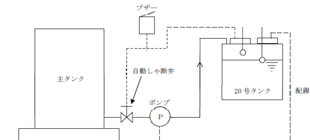
第 3 -17 図 複数の液面感知センサーを設置する例 1
