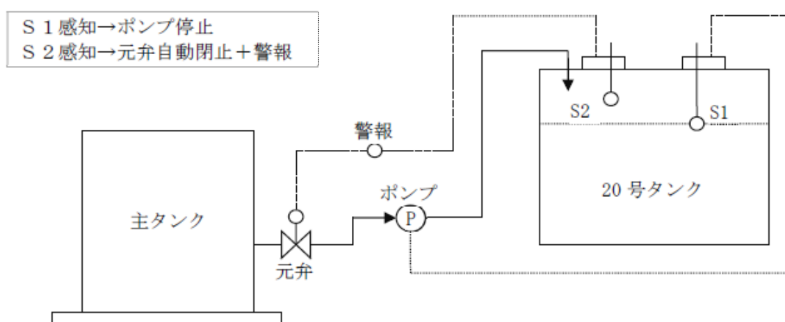
第3 -11 図 液面感知センサーで危険物注入用ポンプを停止させる設備と主タンク（供給元タンク）の元弁を閉止する設備を設置する例
