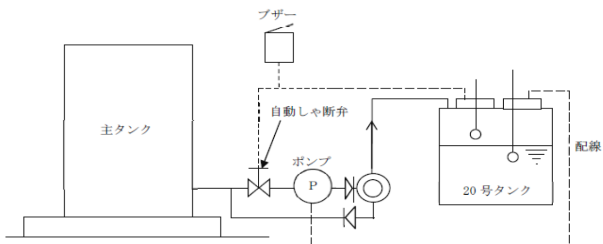
第3 -18 図 複数の液面感知センサーを設置する例2
