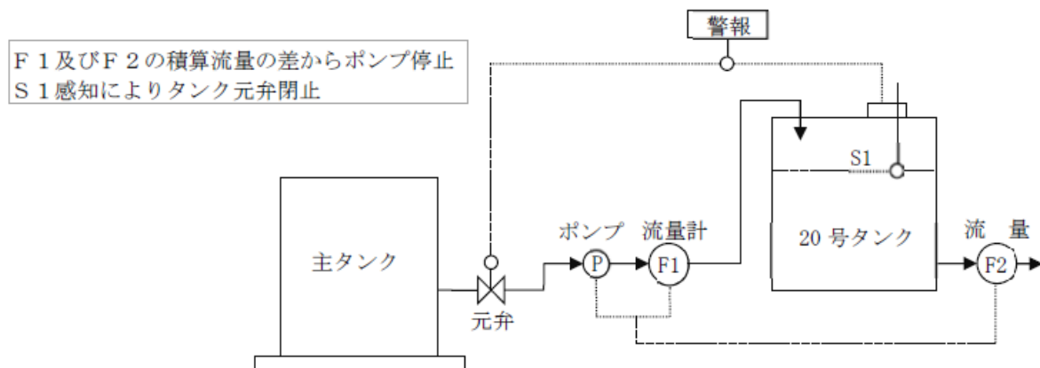
第3-13図 積算流量差を算出し危険物注入用ポンプを停止させる設備と液面感知センサーで元弁を閉止する設備を設置する例
