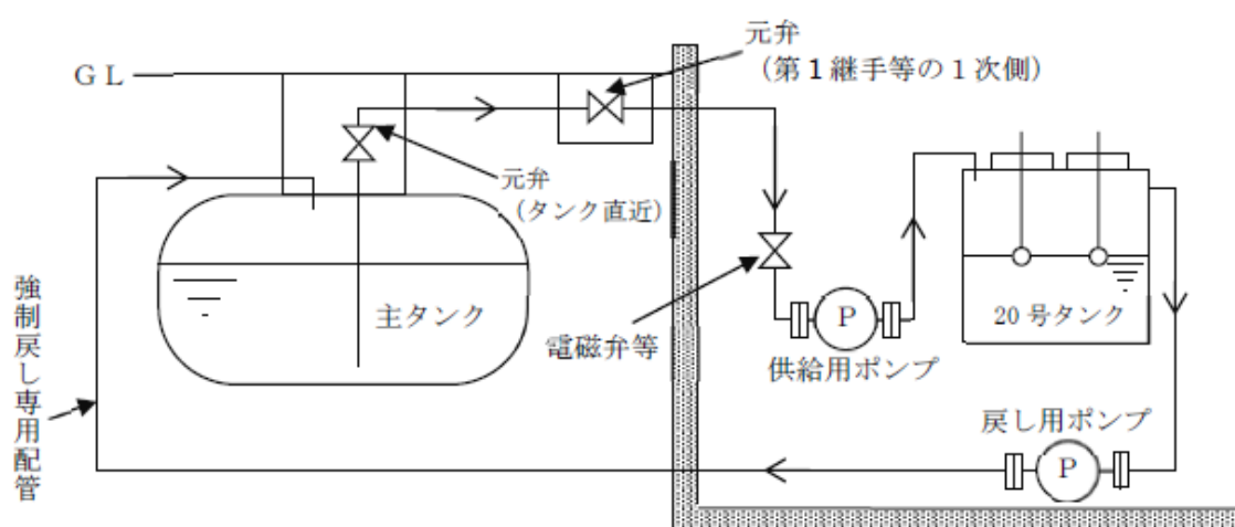
第3 -21 図 配管系等の安全措置（元弁）を設置する例
