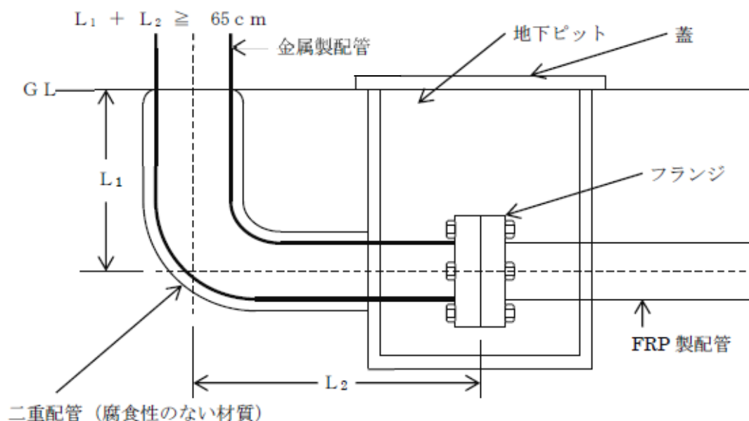
第3-25 図 地下ピット内での接続例
