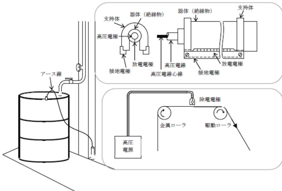
第3-4図 静電気除去装置の設置例
