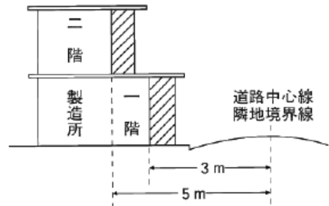
延焼のおそれのある範囲の例
