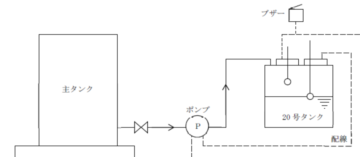
第3 -19 図 複数の液面感知センサーを設置する例3
