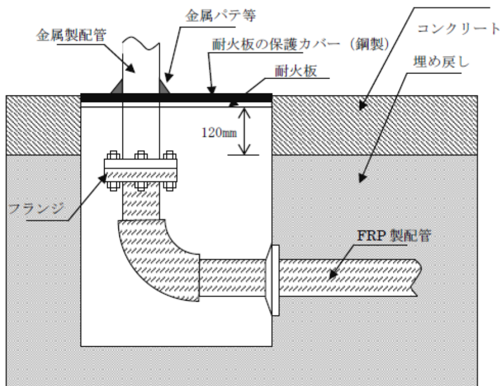
第3 -26図 地下ピット内での接続例2
