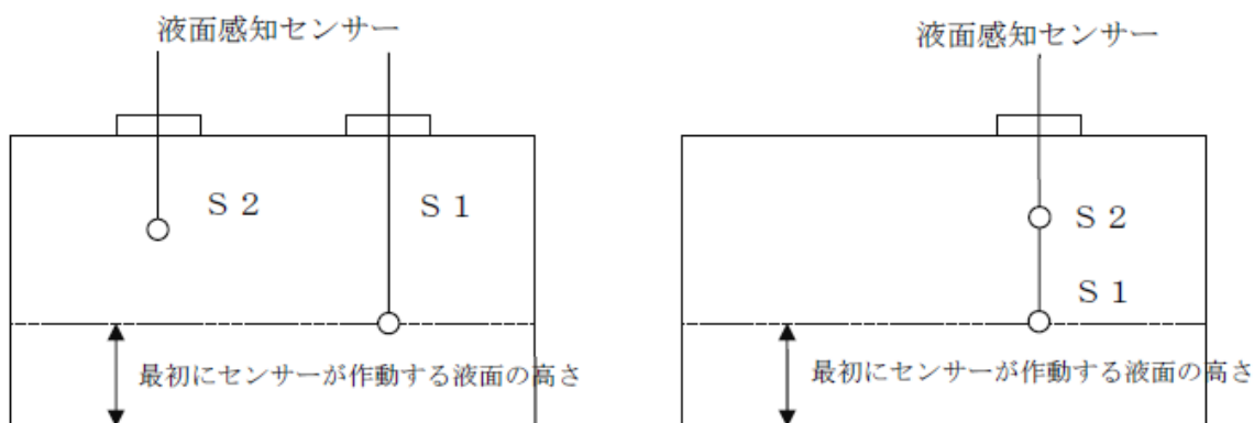
第3-7図 液面感知センサーを設けた20号タンクの液面算定
