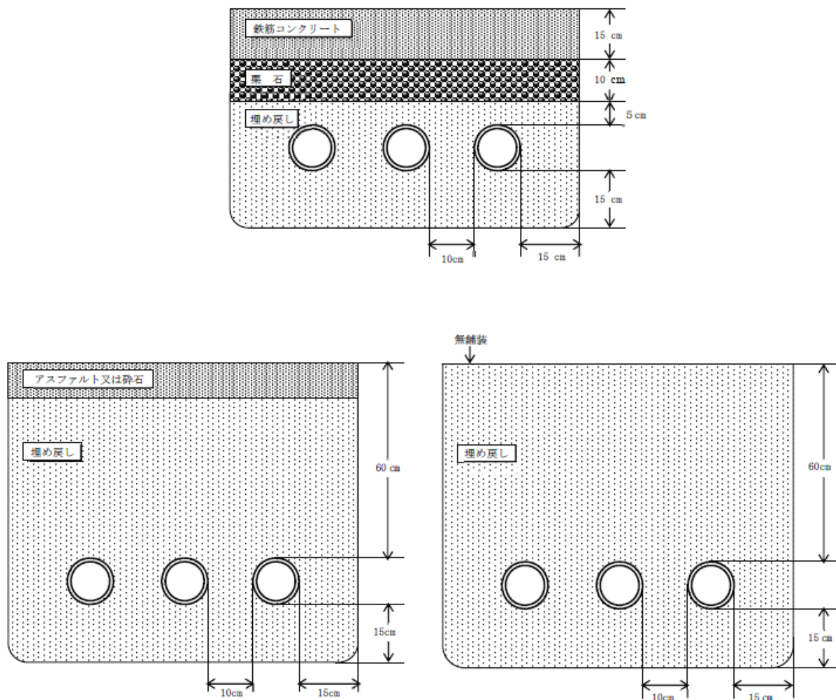
第3 -27図 配管の埋設構造例
