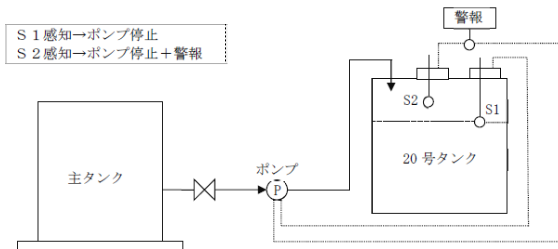
第3 -10 図 液面感知センサーで危険物注入用ポンプを停止させる設備を複数設置する例
