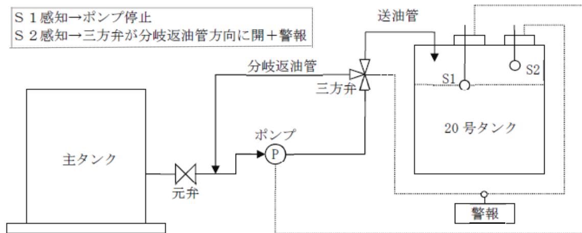
第3-12 図 液面感知センサーで危険物注入用ポンプを停止させる設備と三方弁を制御することで一定量以上の危険物の注入を防止する設備を設置する例
