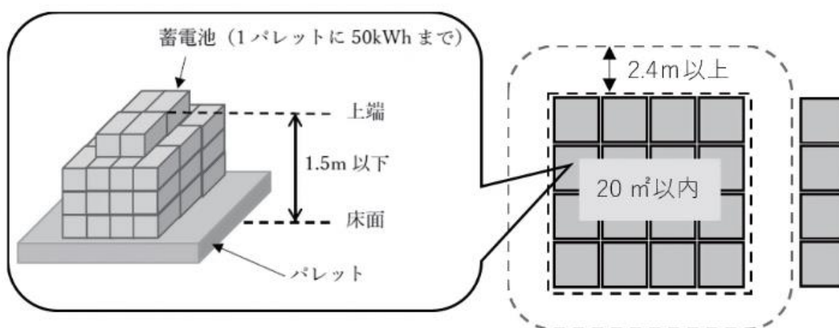
第5-1図 危規則第16条の2の8第2項第5号ハの貯蔵方法の例
