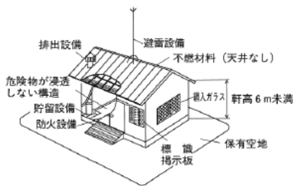
屋内貯蔵所の一般的な構造例
