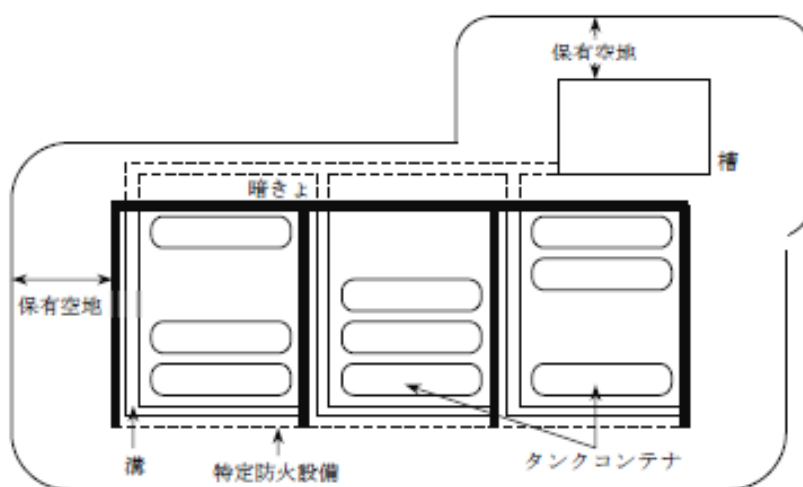
第5-2図 アルキルアルミニウム等をタンクコンテナに収納して貯蔵する屋内貯蔵所
