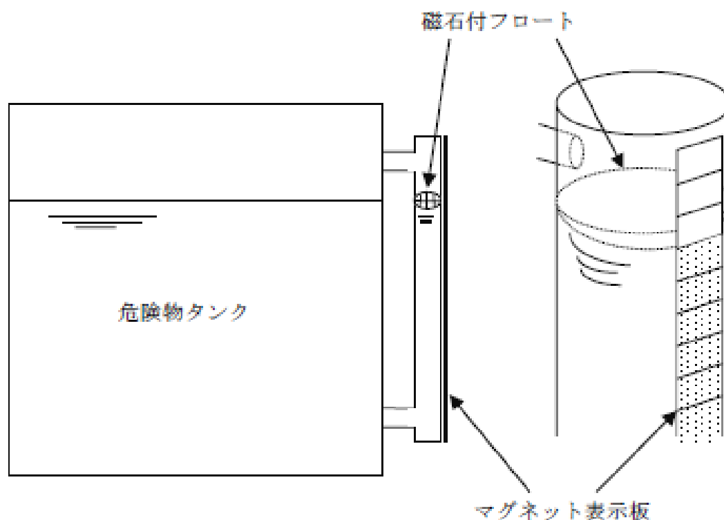
第 6 - 2 図 連通管式自動表示装置の例
