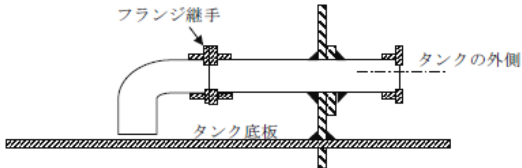
第6－3図 フランジ継手を水抜管のタンク内側部分に取付けた構造例
