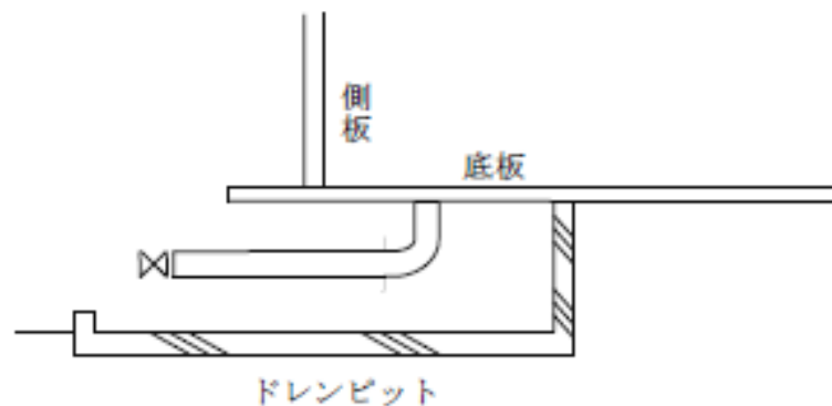
第6-5図 認められない例
