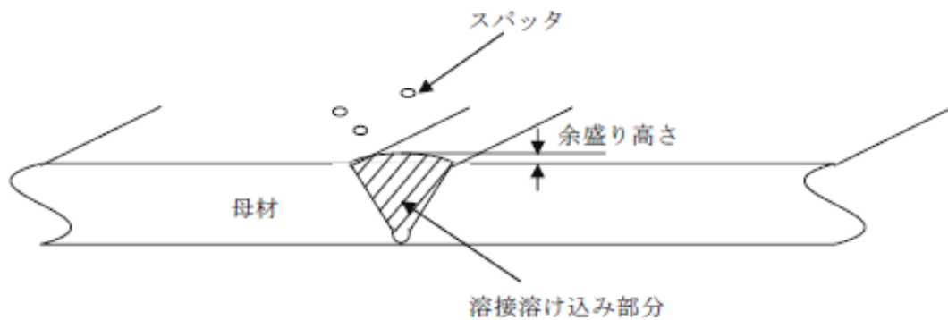
第8－16図 スパッタ等の例
