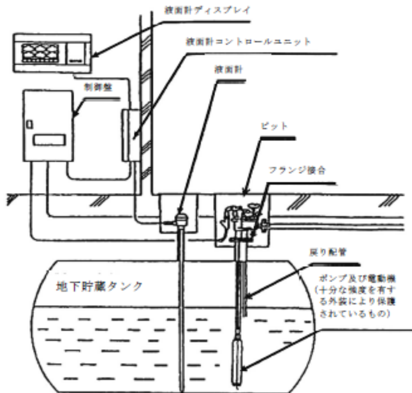
第8-1図 油中ポンプ設備の設置例
