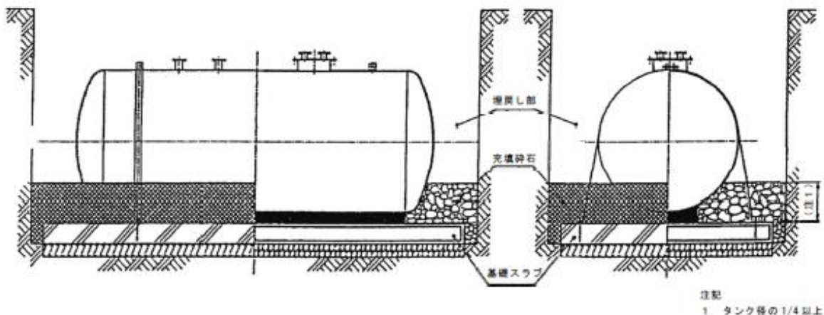
第 8-24 图 充填碎石施工图
