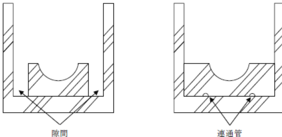
第 8－10 図 タンクからの危険物の漏えいを有効に検知することが可能な構造の例
