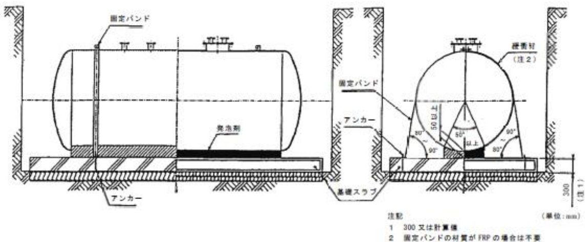
第 8-23 図 発泡材施工図
