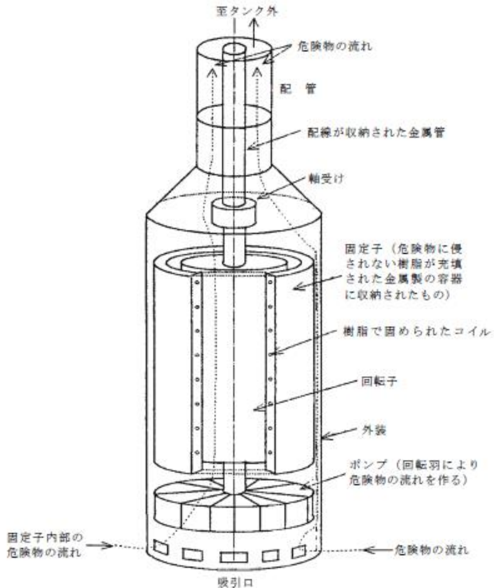
第 8 - 2 図 油中ポンプ模式図
