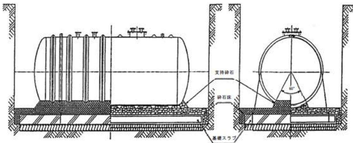
第 8 - 19 図 支持碎石施工図
