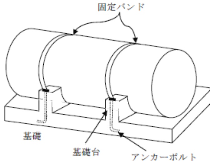
第8-15図 タンクの固定方法
