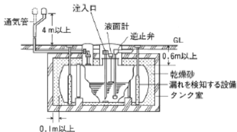
タンク室方式による設置の例
