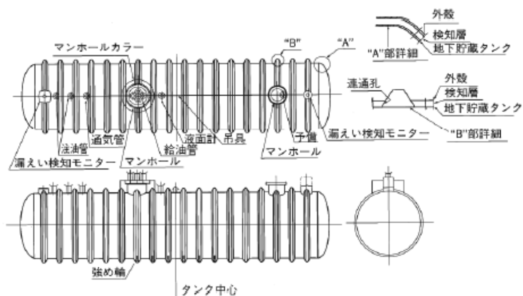
強化プラスチック製二重殻タンクの構造例 (FF 二重殻タンク)
