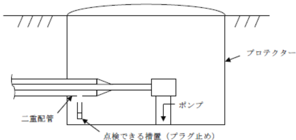
第 8－3 図 容易に漏れいが点検できる措置の例
