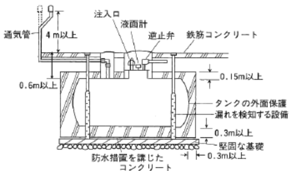
危険物の漏れ防止構造による設置の例
