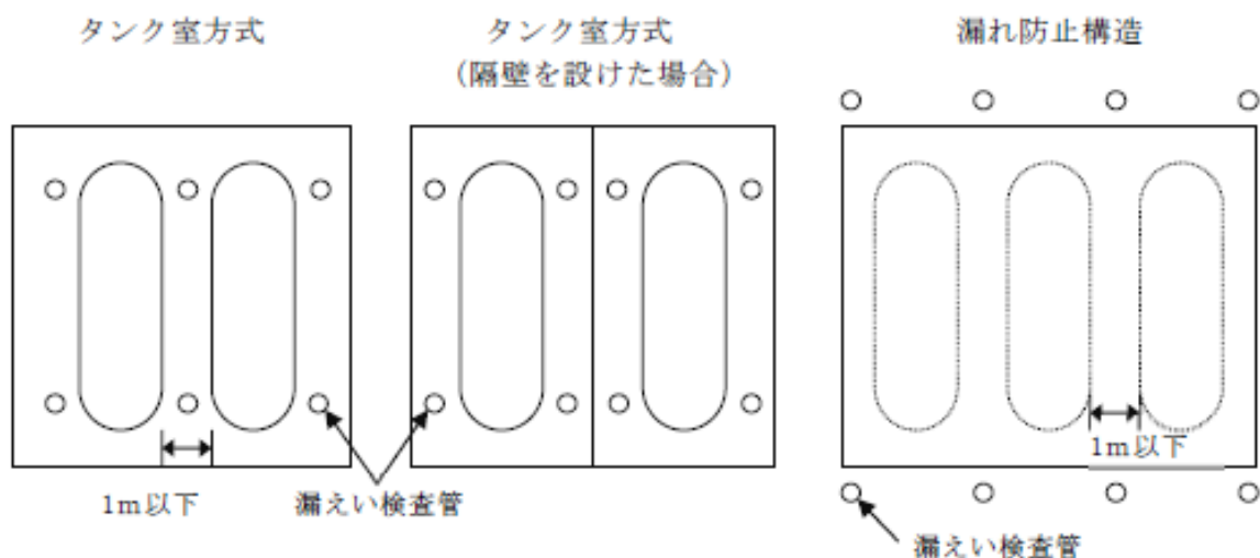
第 8 - 5 図 漏えい検査管の設置例
