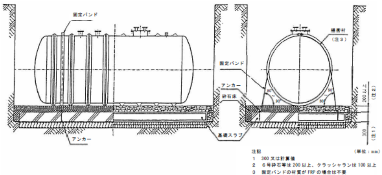
第8-18図 砕石床施工図
