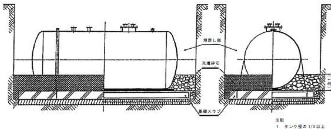
第8-22図 充填碎石施工図 (支持碎石は、第8-19図のとおり施工されているものとする。)
