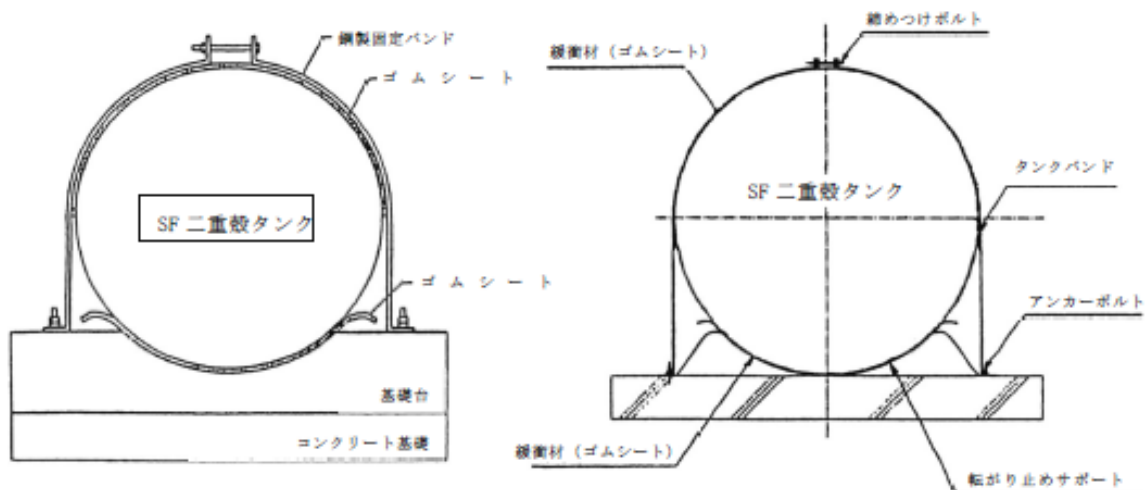
第8－17図 接触面の保護措置の例
