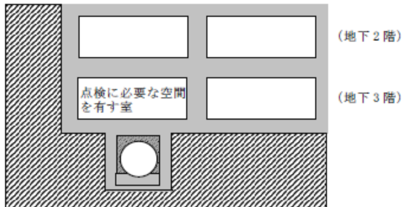
第8－6図 建物の下部にタンク室を設ける例
