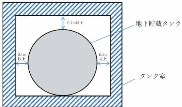
第 8－25 図 タンクの底部とタンク室の内側との間隔を 0.1 メートル未満とした場合の例
