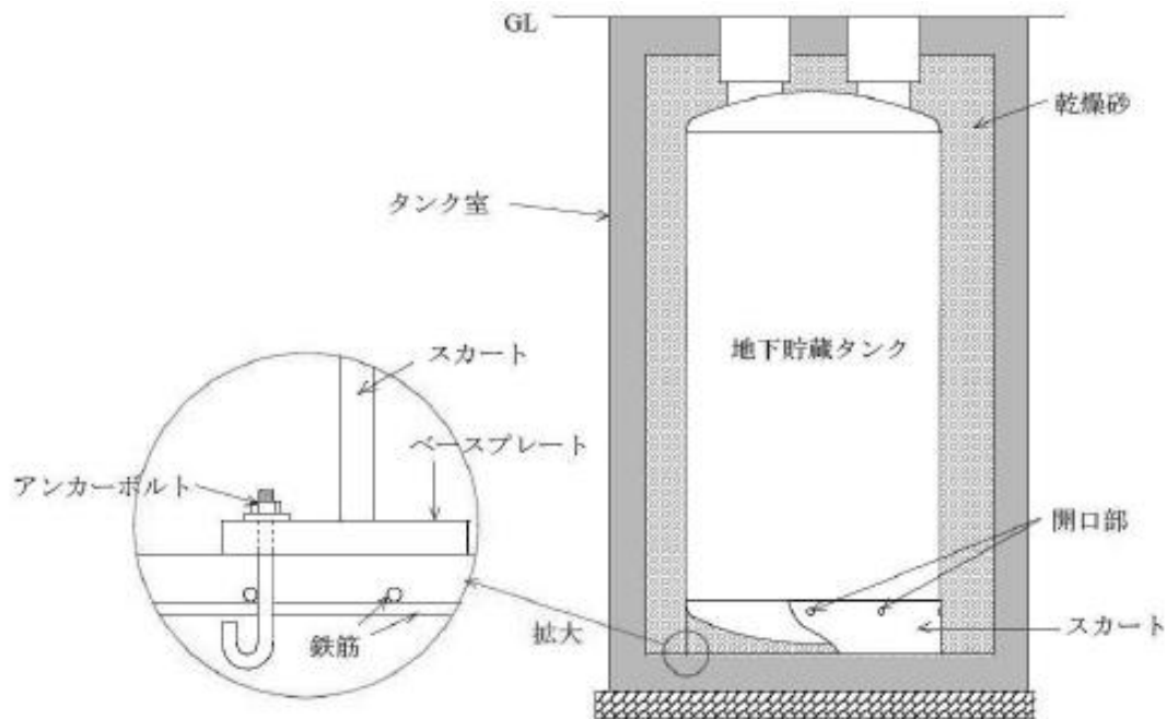
第 8-12 図 横置円筒型地下貯蔵タンク以外のタンクである縦置円筒型地下貯蔵タンクの例
