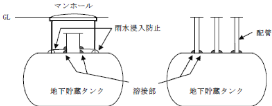
第8－4図 配管類の取り付け方法
