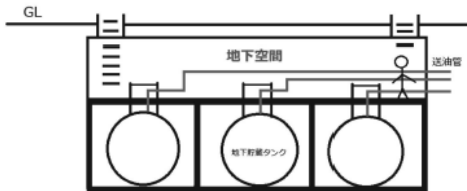
第8－7図 タンク室上部と地盤面の間の地下空間
