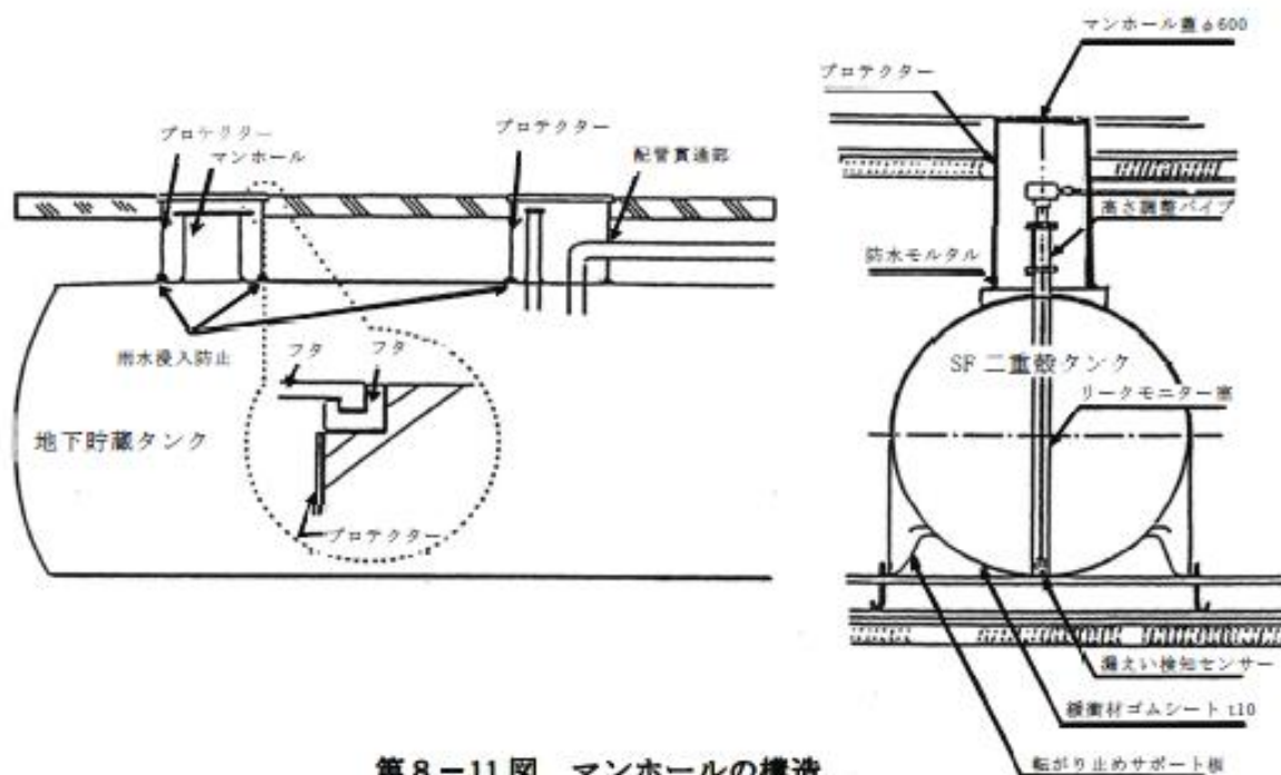
第 8-11 図 マンホールの構造
