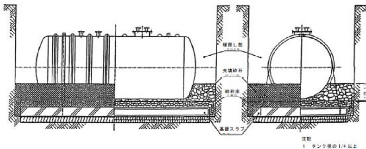
第 8 - 20 図 充填碎石施工図
