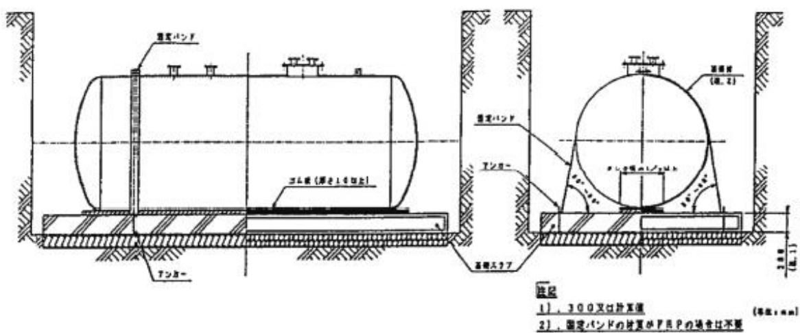
第8-21図 ゴム板施工図
