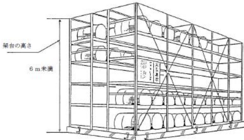
第11-1図 架台の高さ
