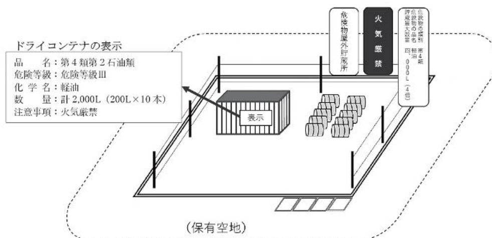
第11-2図 軽油をドライコンテナ（ドラム缶（10本））とドラム缶（10本）で貯蔵する場合のイメージとコンテナの表示
