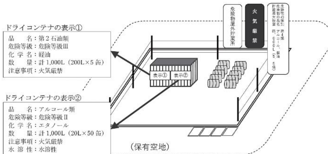
第11-3図 ドライコンテナにより軽油（ドラム缶（5本））とアルコール（20L×50缶）を貯蔵し、ドラム缶（10本）で軽油を貯蔵する場合のイメージとコンテナの表示
