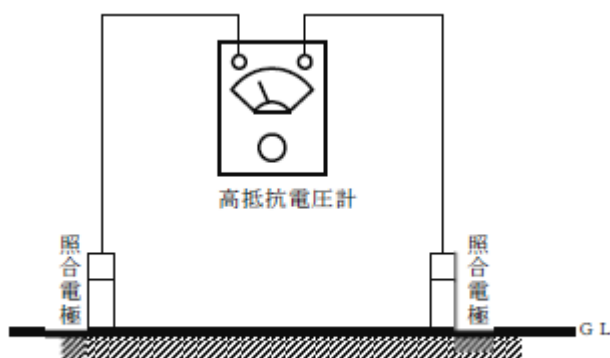
第14-2図 地表面電位こう配測定方法
