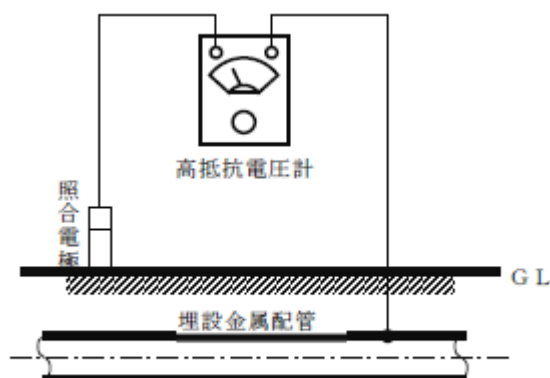
第14-1図 対地電位測定方法
