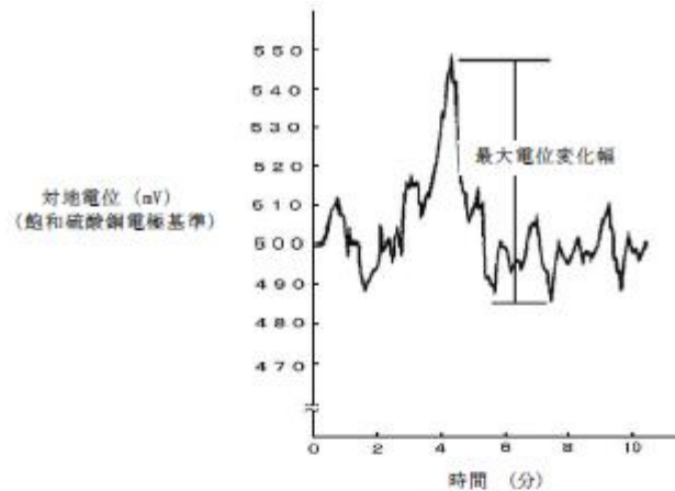
第14-3図 対地電位測定例
