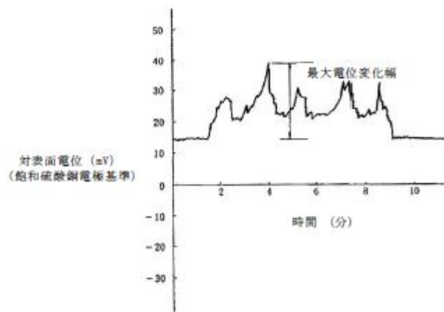
第14-4図 地表面電位
