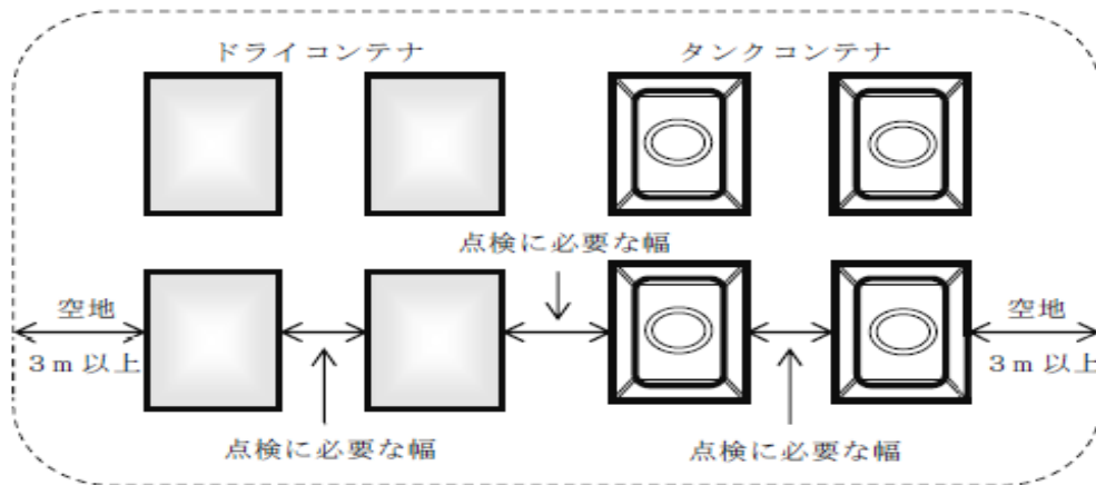
第2-1図 タンクコンテナとドライコンテナを同一の場所に仮貯蔵する例
