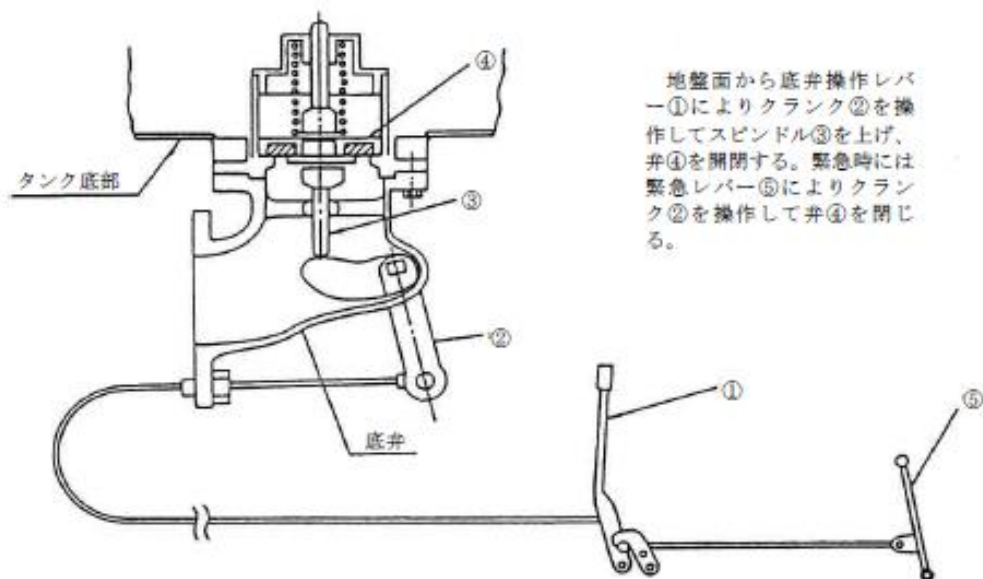
例 2 - 1 地盤面上において底弁を開閉する構造のもの
