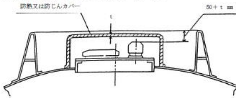
例 1 内側に断熱材が張り付けられていないもの
