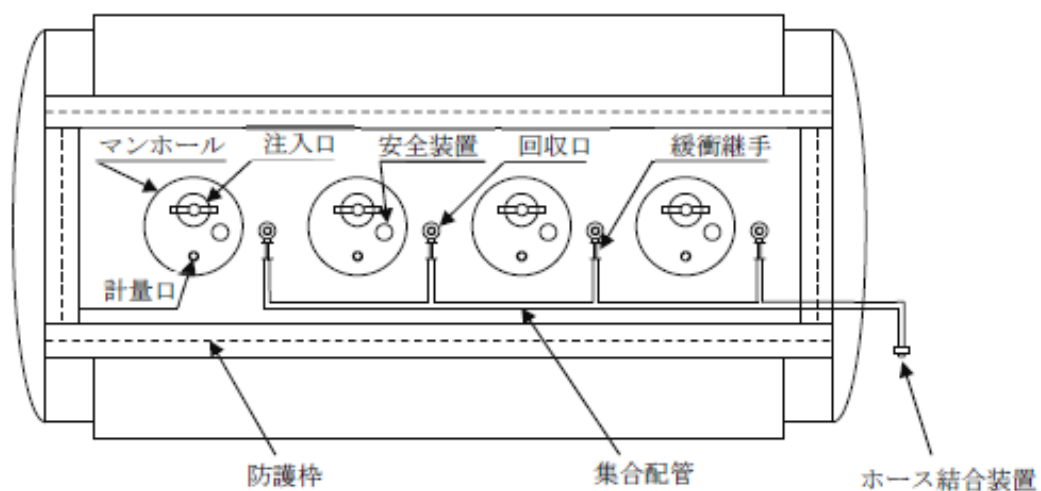
第 10-10 図 集合配管の取り付け例
