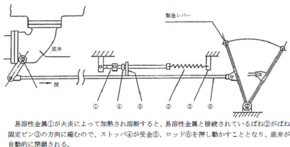
第 10—35 図 自動閉鎖装置の構造例
