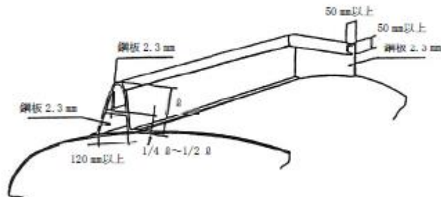
第10-26図 防護枠の構造
