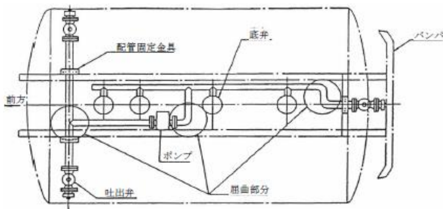
第10-39図 配管による方法
