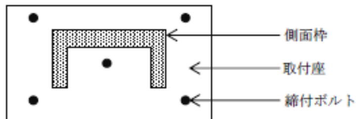
第10－23図 締付ボルト配列の例
