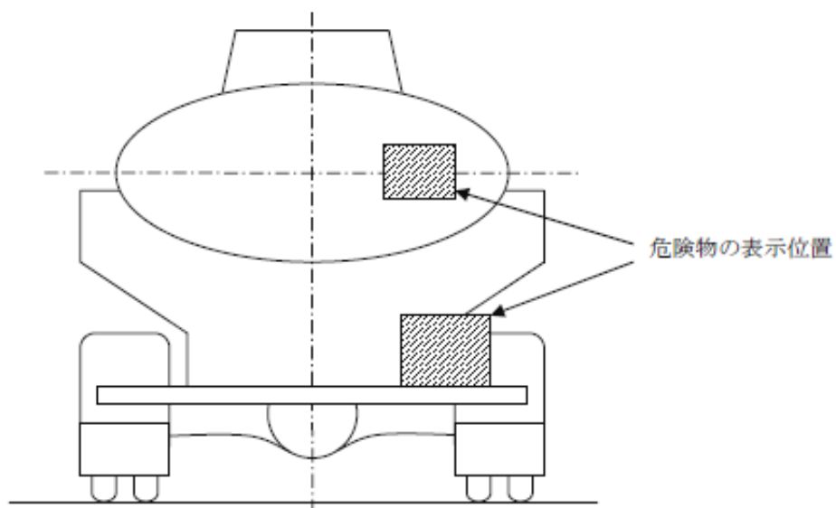
第10-48図 表示の位置
