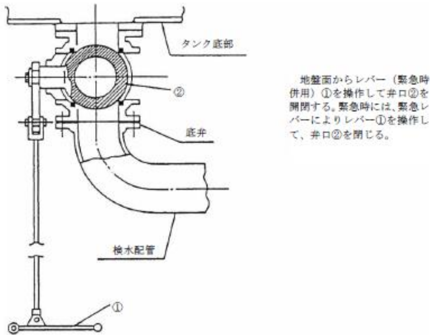
第 10－32 図 底弁の構造例
