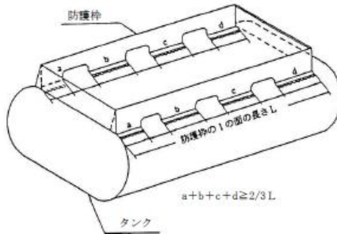
第 10-30 図 防護棒とタンク胴板との間の溶接線の減少例 (断熱効果を良くするため防護棒の溶接部を減少した例)
