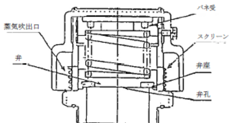
第10-4図 安全装置の構造例
