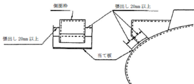
例1 箱形の側面枠に設ける当て板
