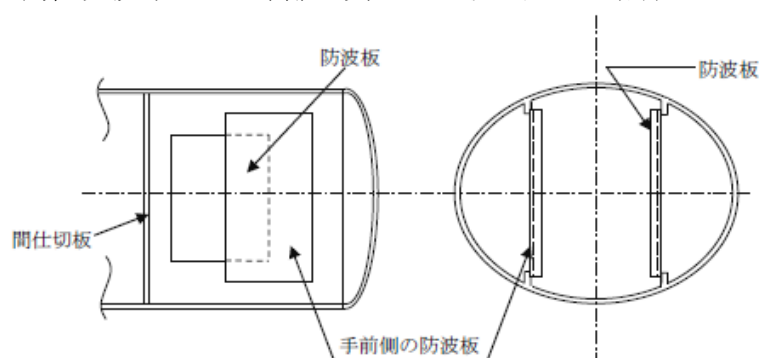
第10-6図 防波板の取付方法
