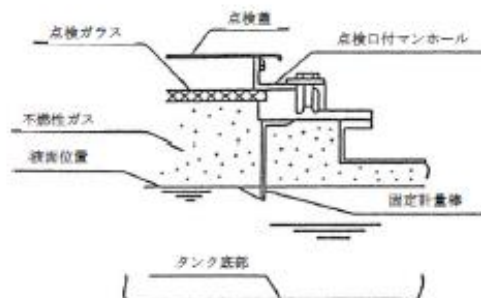
例8 不燃性ガスを封入した状態の ままで計量でき、計量棒がタン ク底部と接触しなくてもよい例
