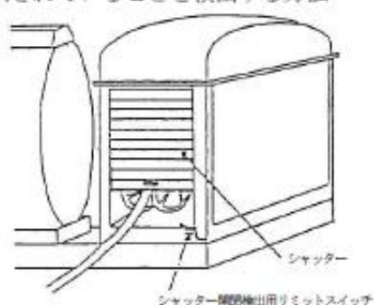
第10-66図 給油設備の扉による方法の例
