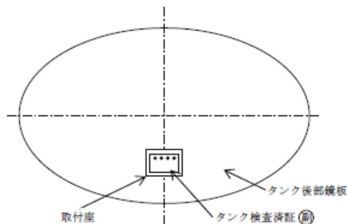
第 10-73 図 タンク検査済証 (副) 取付位置
