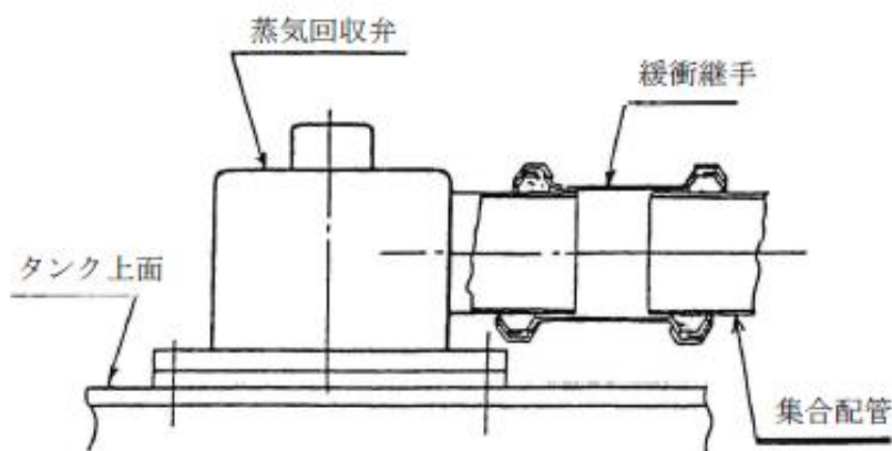
例2 緩衝継手を使用した例
