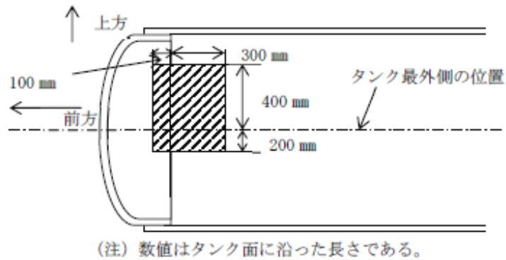
第10-3図 タンク本体の応力集中防止の範囲
