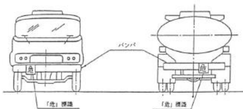
第 10-51 図 標識の取付位置
