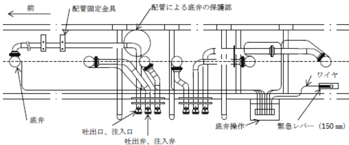
第 10-56 図 ボトムローディング配管の例 (片側)
