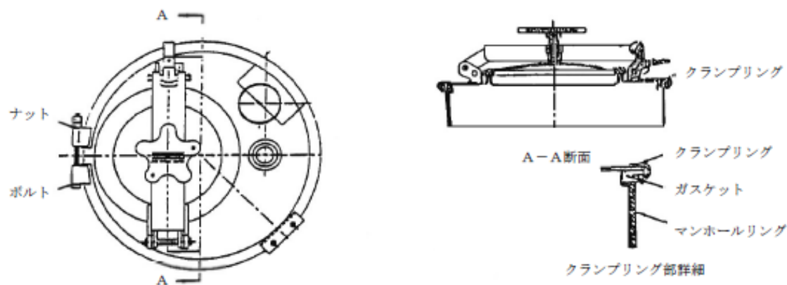
第10-7図 クランプリング方式のマンホールカバーの例
