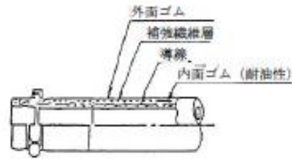
第10-70図 静電気を導通させる給油ホースの例
