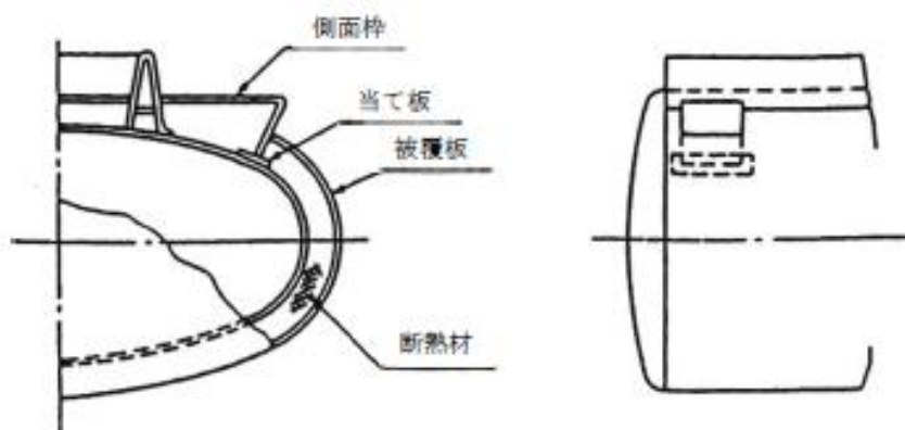
第 10-21 図 タンク胴板に直接取り付ける側面杵の例
