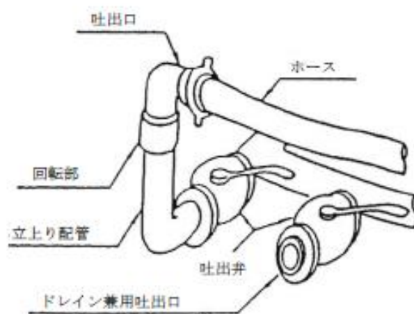
第 10-46 図 配管先端部の構造例
