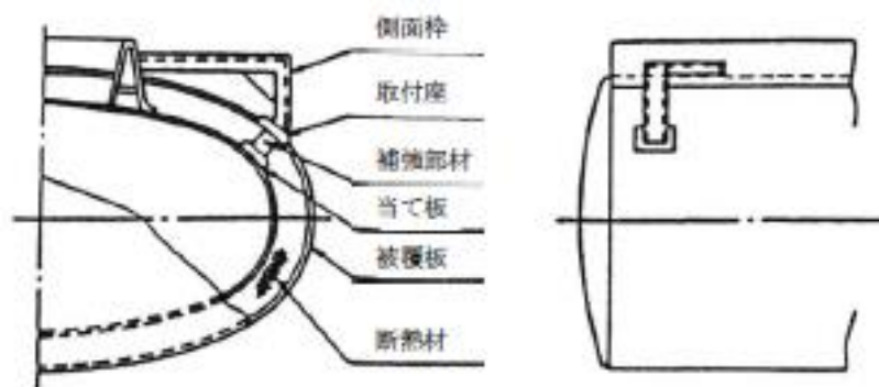
第 10-19 図 外板の下部に補強部材を設ける側面枠の例 (側面枠と補強部材とを溶接接合する場合)
