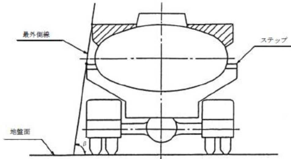
例3 側面枠頂点とタンク側面とを結んだ例
