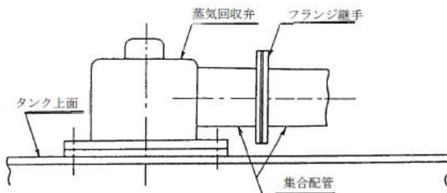
例1 フランジ継手を使用した例
