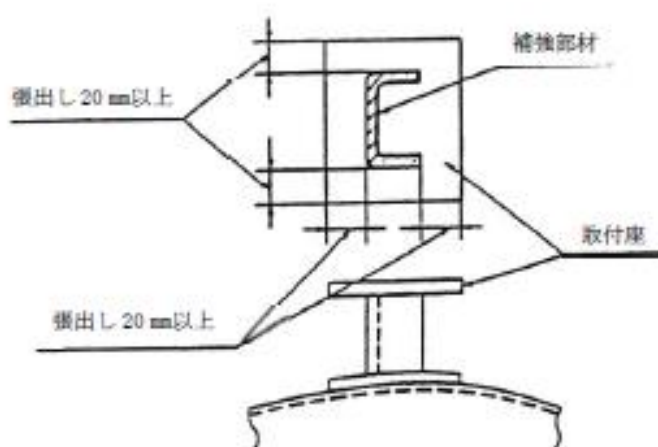
第 10-22 図 取付座の大きさ
