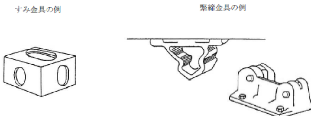
第10-57図 JISにより造られた緊締金具及びすみ金具の例
