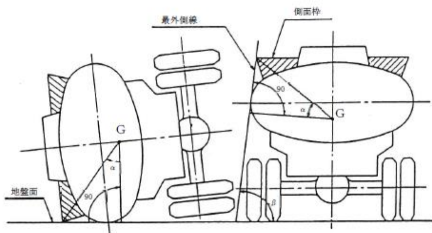
第10-17図 側面枠取付図
