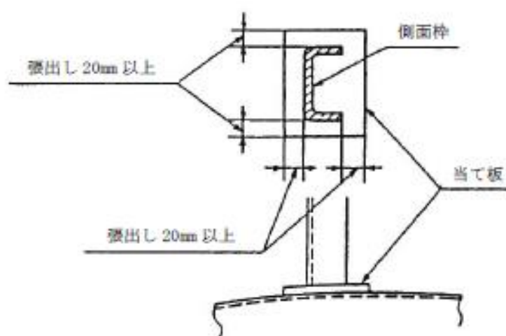
第10-15図 当て板
