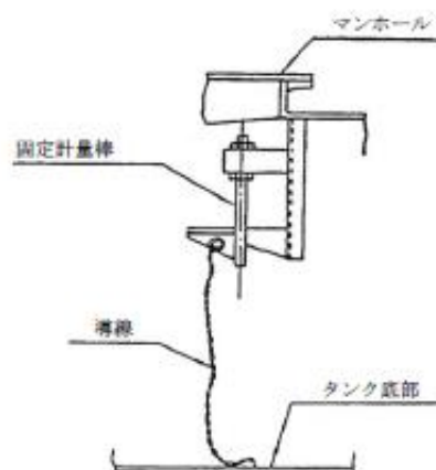
例6 固定計量棒に導線を取り 付ける例
