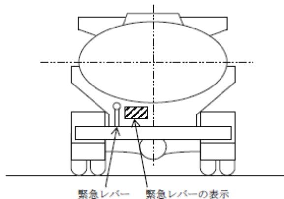
第10-37図 緊急レバーの表示位置の例
