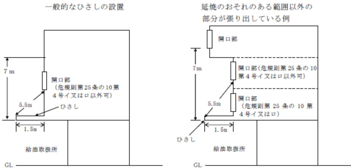
第12・49 図 延焼防止上有効な屋根又はひさしの設置例
