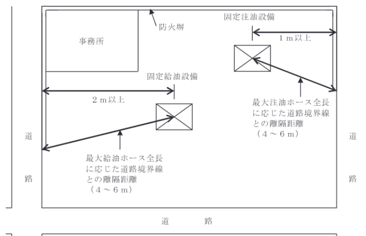
第12-2図 固定給油設備等の位置（例）
