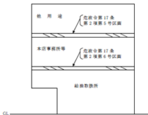
第12-43 図 上部に上階がある場合の判定例。
