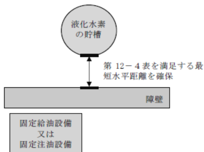
第 12-62 図 障壁から必要な最短水平距離を確保する方法
