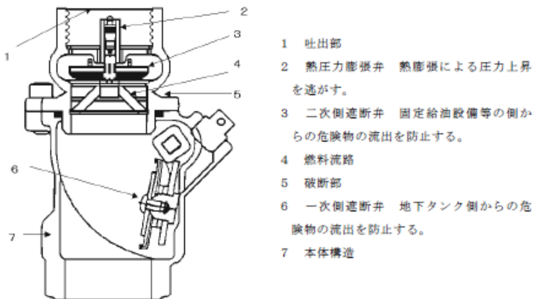
第12-74 図 立ち上がり配管遮断弁の構造例
