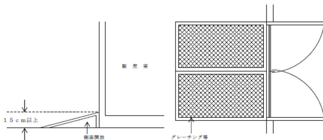
第12-20図 可燃性蒸気滞留防止構造例
