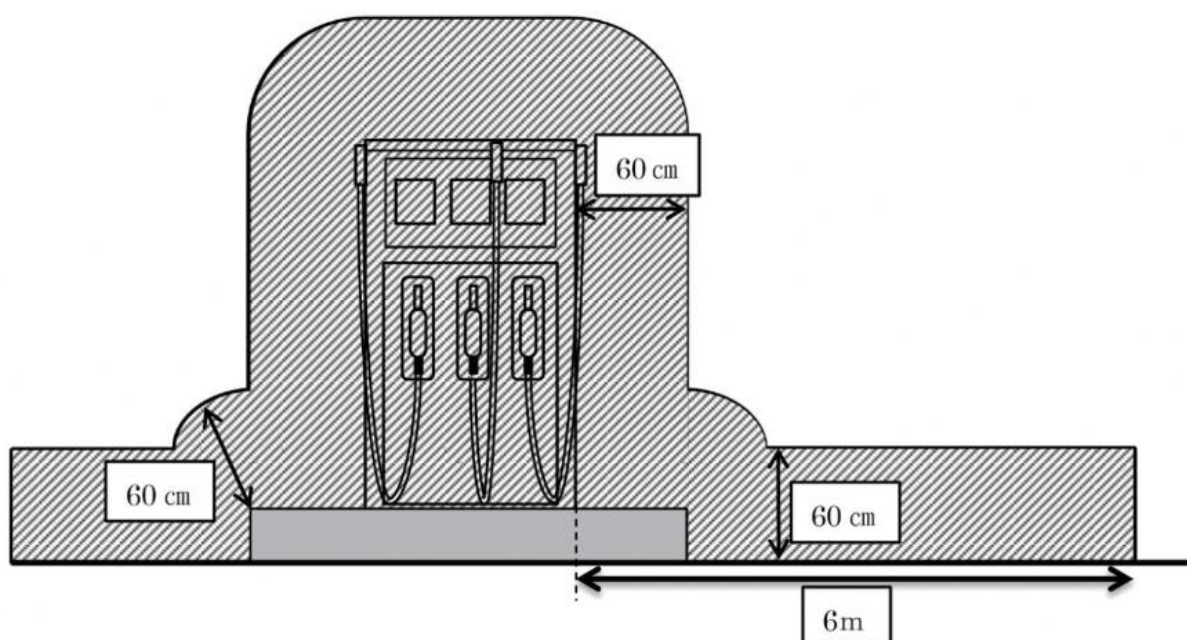
第 12-31 図 固定給油設備の周囲で可燃性の蒸気が滞留するおそれのない場所（斜線部分以外）
