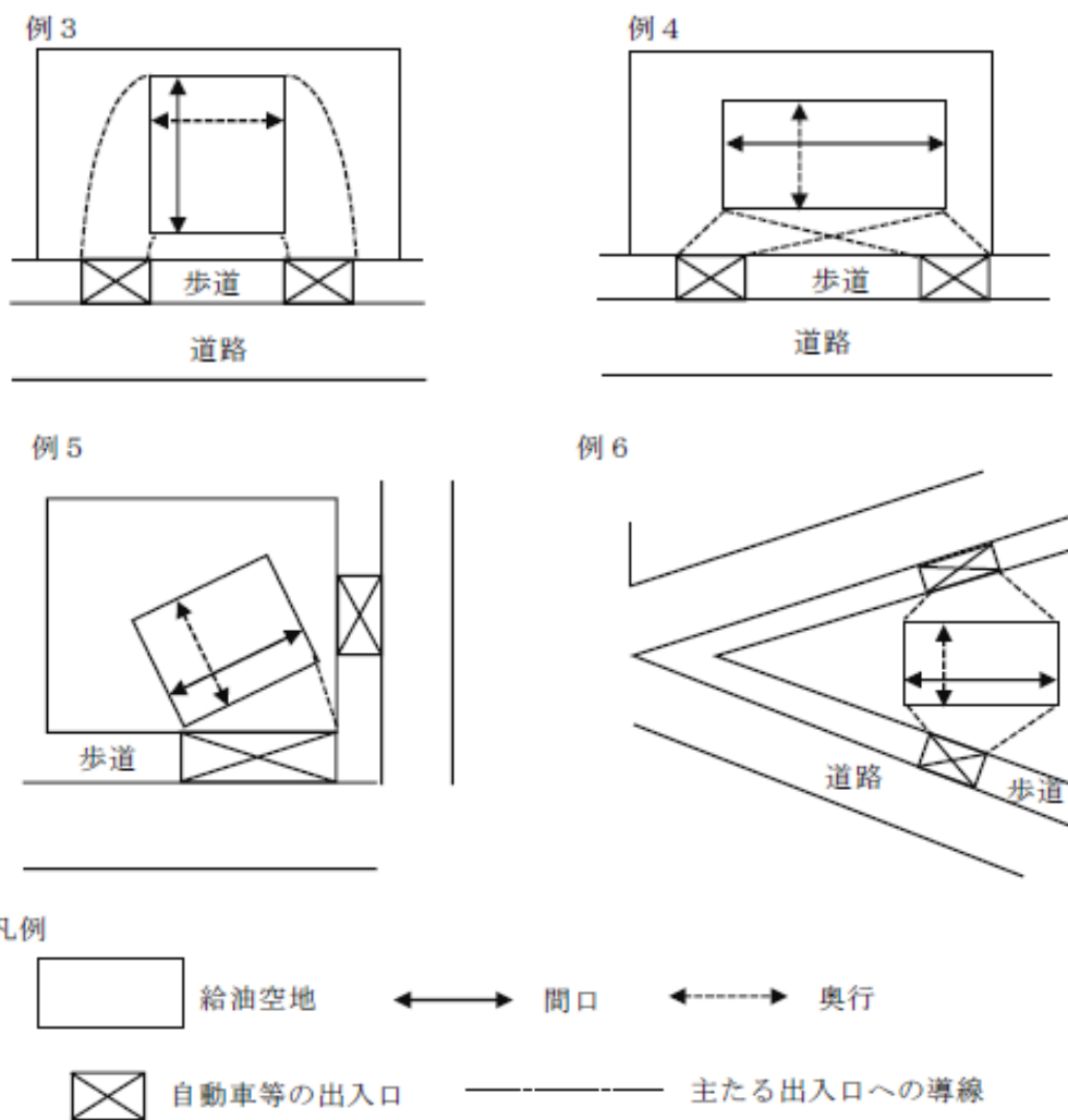
第 12-25 図 給油空地の例図
