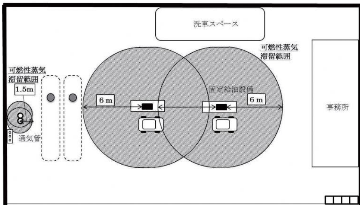
第 12-34 図 給油取扱所（平面図）で可燃性の蒸気が滞留するおそれのない場所（斜線部分以外）
