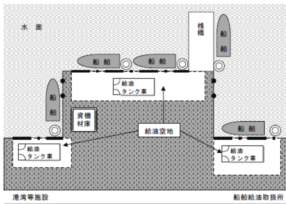
第 12- 51 図 一の船舶給油取扱所内に複数の給油空地を設ける場合の設置例
