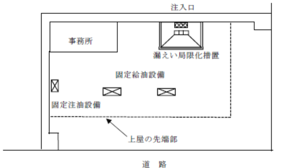
第 12-46 図 注入口及び固定給油設備等の上階への延焼防止上安全な場所
