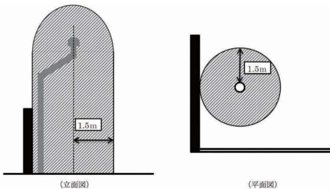
第 12-33 図 通気管の周囲で可燃性の蒸気が滞留するおそれのない場所（斜線部分以外）
