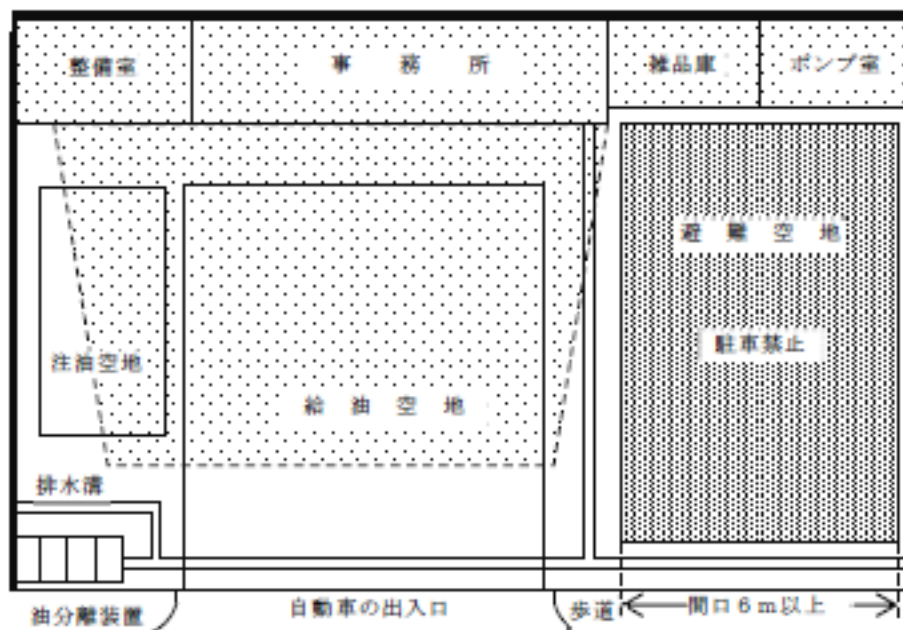
第 12-40 図 避難空地
