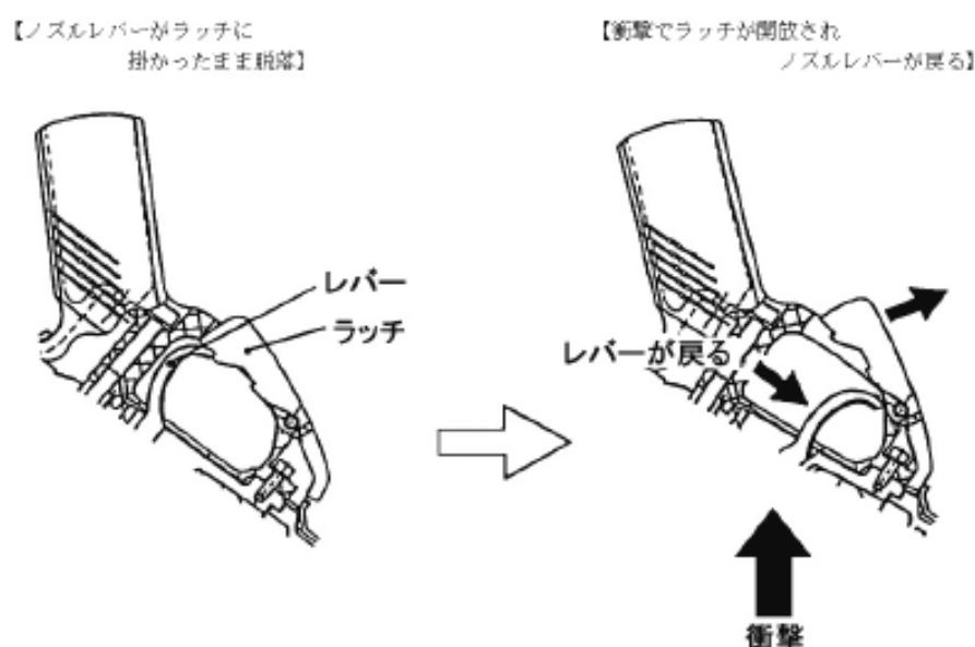
第12-71 図 脱落時停止制御装置の作動例
