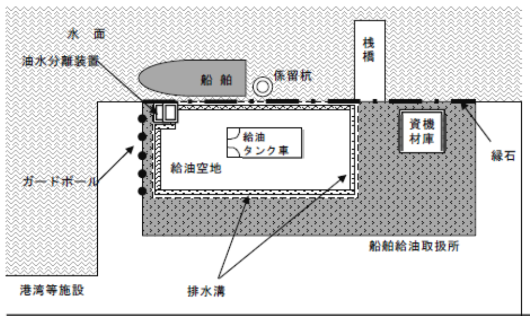
第 12- 50 図 船舶給油取扱所の設置例
