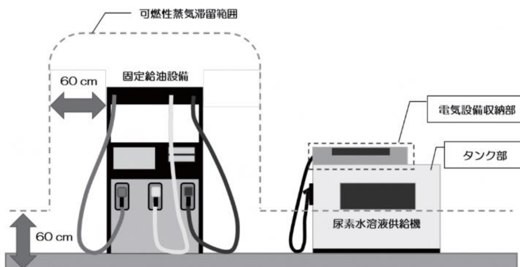
第 12-29 図 尿素水溶液供給機の設置例（電動ポンプにより払い出すタイプ）
