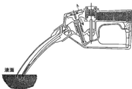
第 12-73 図 滴量停止制御装置の構造例
