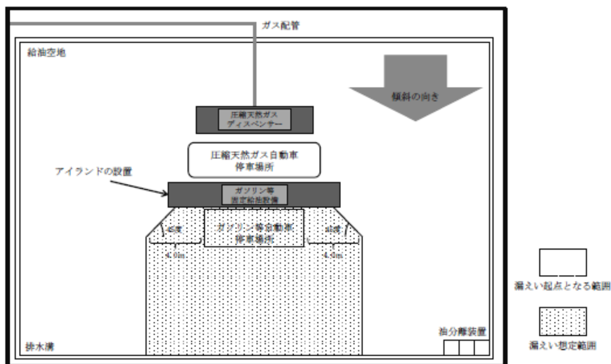
第 12- 60 図 圧縮天然ガススタンドのディスペンサー及びガス配管を給油空地に設置する例 2
