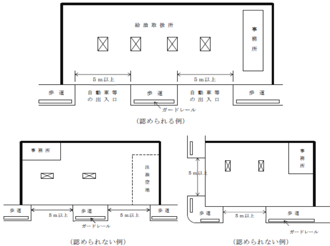
第 12-22 図 自動車等の出入口
