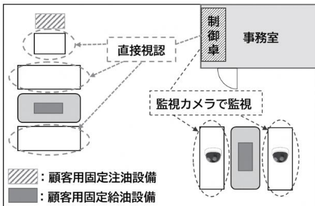
第 12-79 図 認められない制御卓の位置の例
