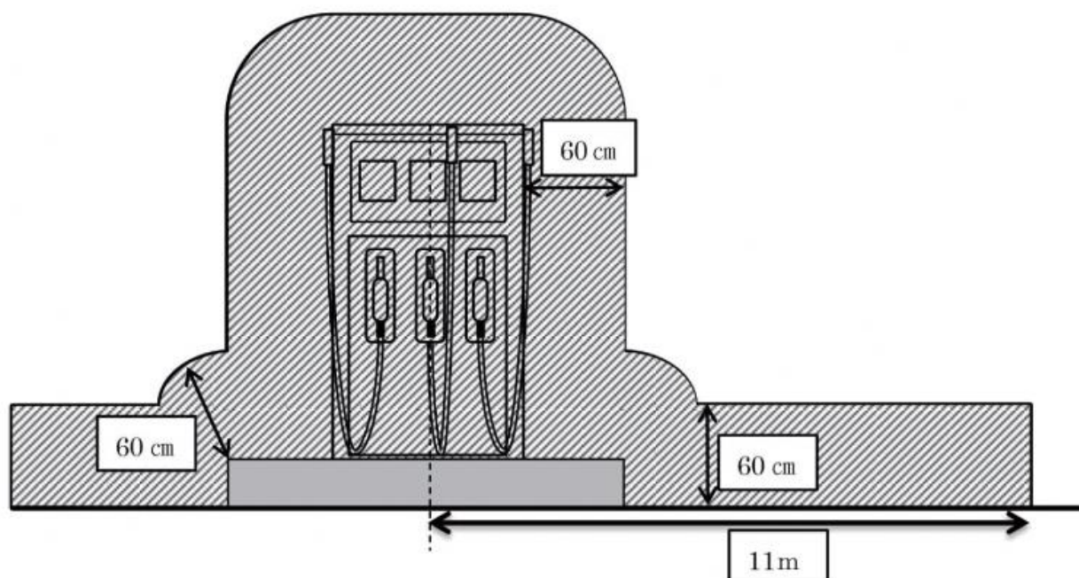
第 12-35 図 固定給油設備の周囲で危険物の流出その他の事故により発生した可燃性の蒸気が滞留するおそれのない場所（斜線部分以外）
