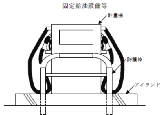
第12-42図 衝突防止措置の例
