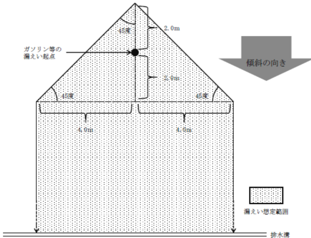
第 12-58 図 検証に基づくガソリン等の漏えい想定範囲
