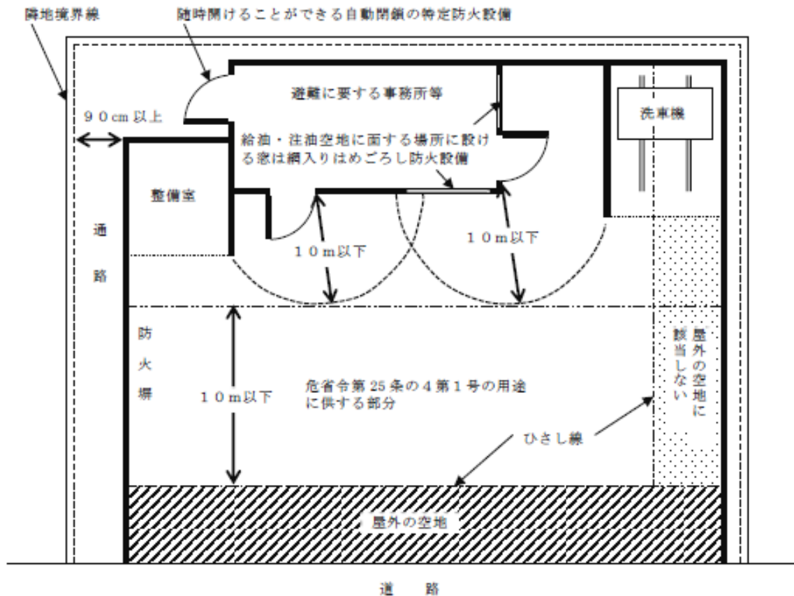
第 12-41 図 避難通路の確保例
