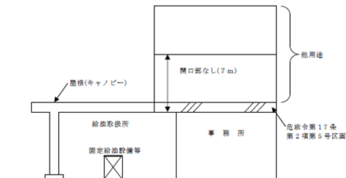
第12-44 図 上部に上階がある場合の屋根（キャノピー）等の構造例。
