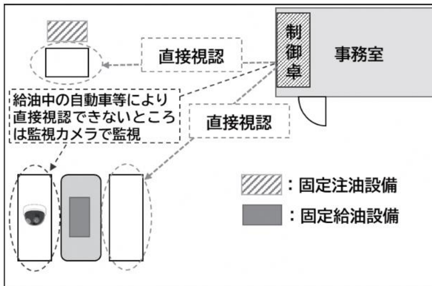
第 12-77 図 全ての顧客用固定給油設備等における使用状況を直接視認できる位置に制御卓を設置する例
