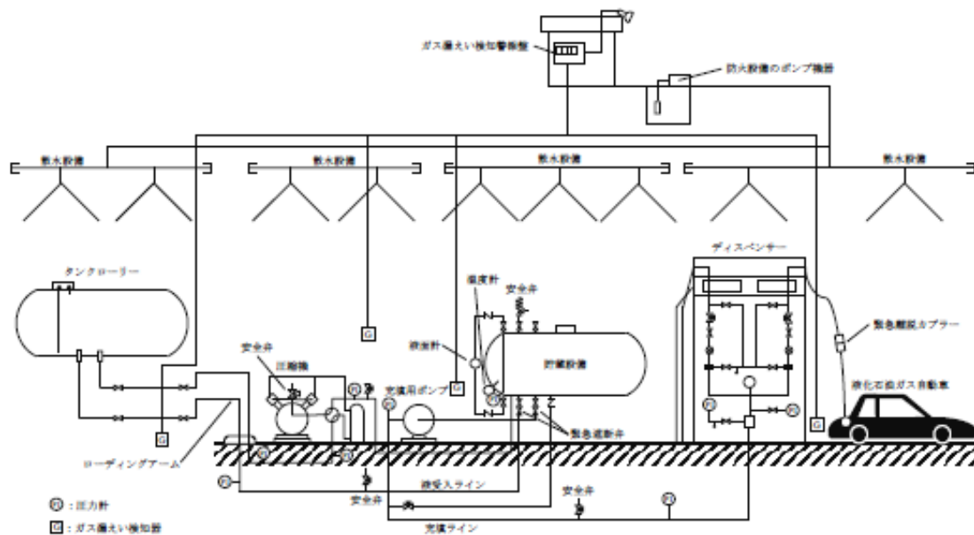
第 12- 56 図 屋外給油取扱所に液化石油ガススタンドを併設した例
