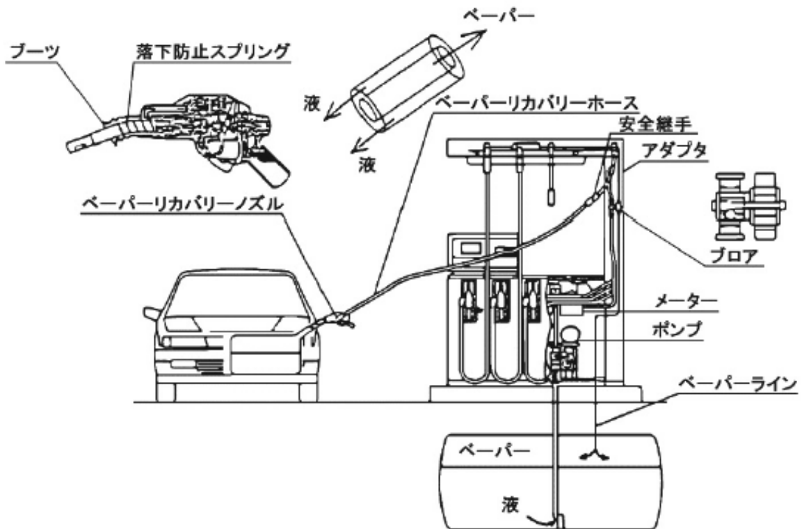
第 12- 72 図 可燃性蒸気回収装置の構造例
