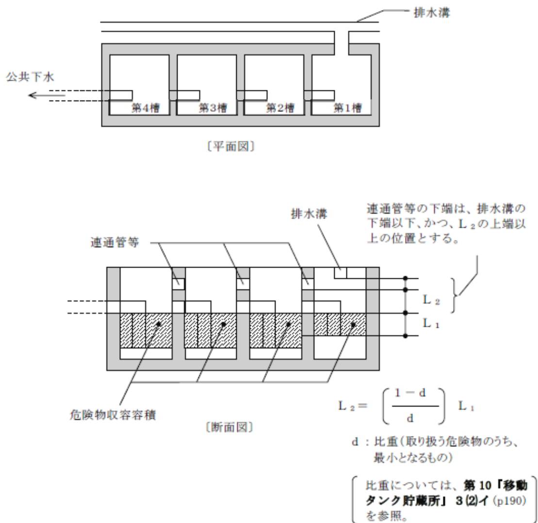
第12-8図 油分離装置の平面図及び断面図（例）
