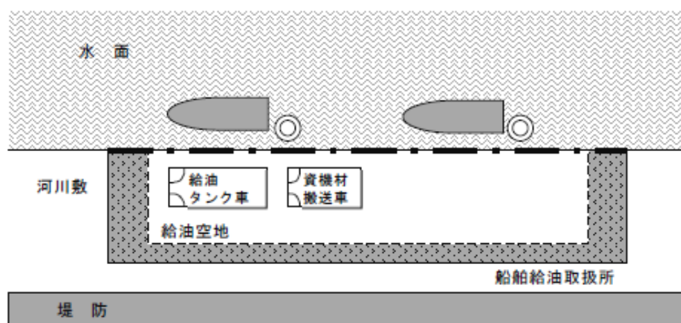
第 12- 52 図 給油時に流出防止設備等の資機材を搬送する場合の設置例
