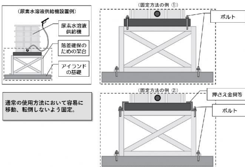
第 12-30 図 尿素水溶液供給機の設置例（重力により払い出すタイプ）
