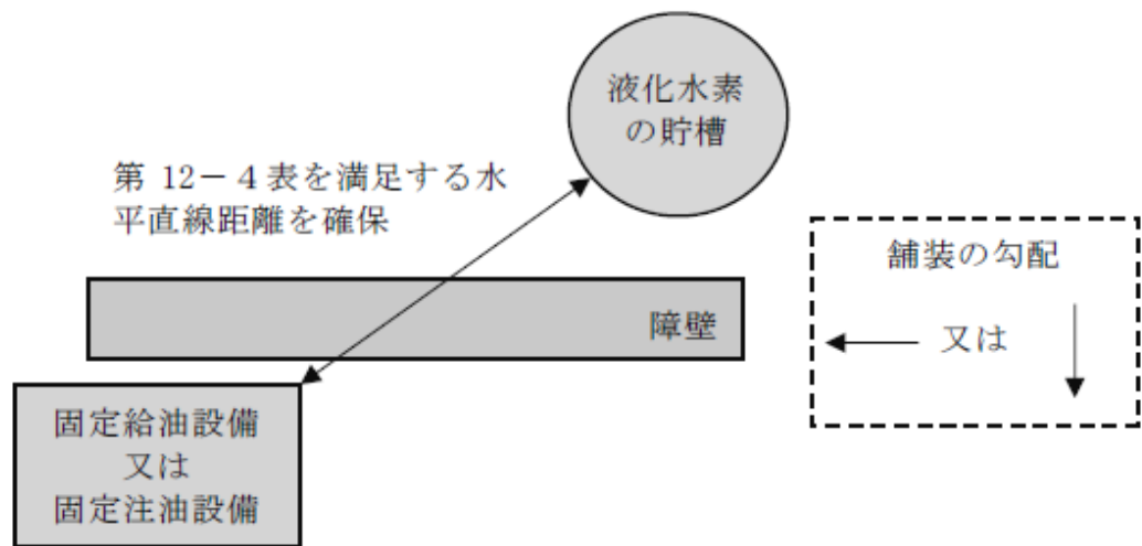
第12-63 図 固定給油設備及び固定注油設備から必要な水平直線距離を確保する方法
