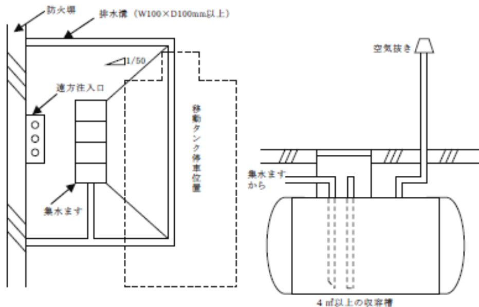
第 12- 48 図 漏えい局限化措置の例
