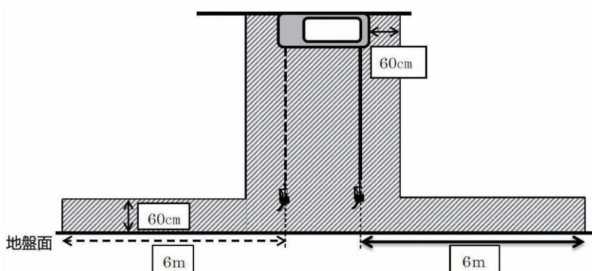
第 12-32 図 懸垂式の固定給油設備の周囲で可燃性の蒸気が滞留するおそれのない場所（斜線部分以外）
