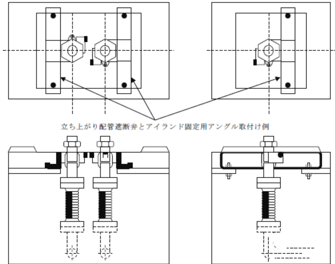
第 12-75 図 立ち上がり配管遮断弁の取付け例
