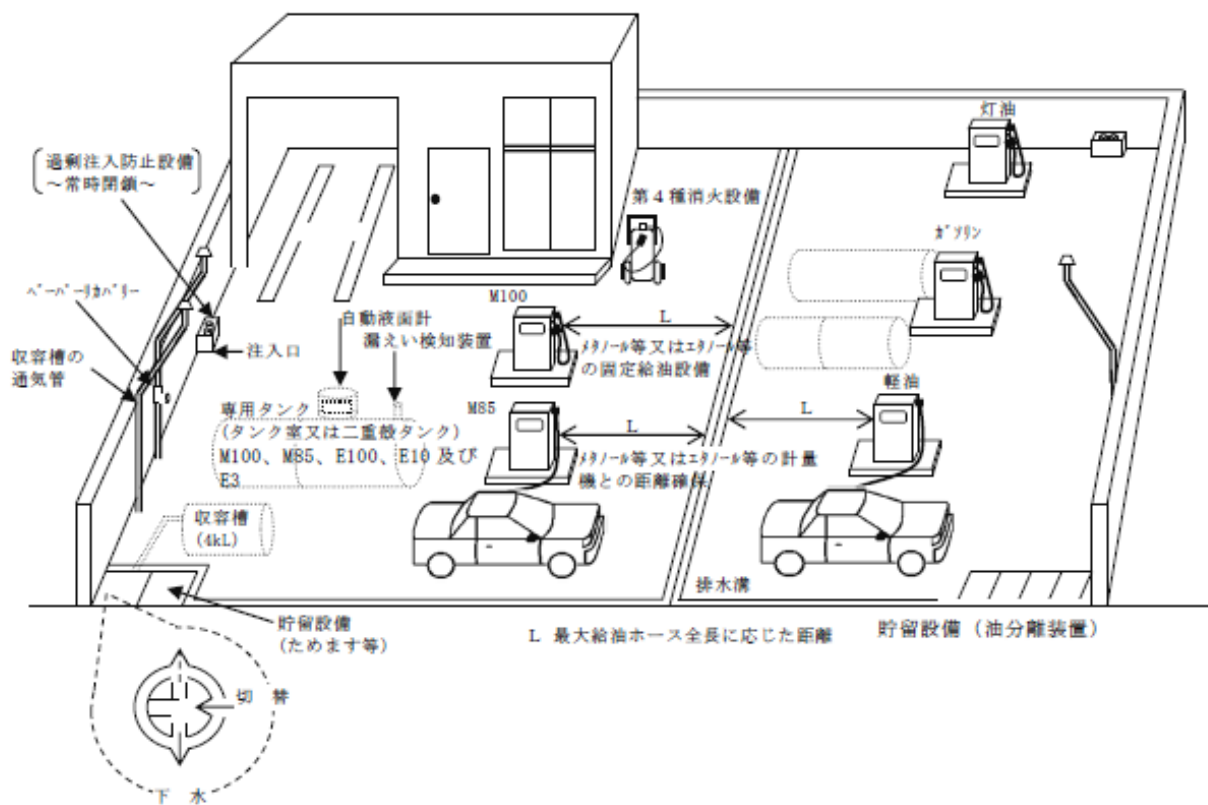
第 12・70 図 ガソリン等とメタノール等又はエタノール等を取り扱う給油取扱所の設置例
