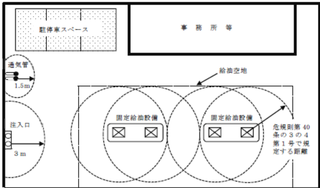
第12-13図 駐停車スペースの例
