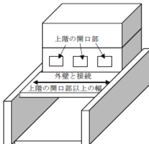
第 12-47 図 上階への延焼防止上有効な幅を有して外壁と接続した屋根の例
