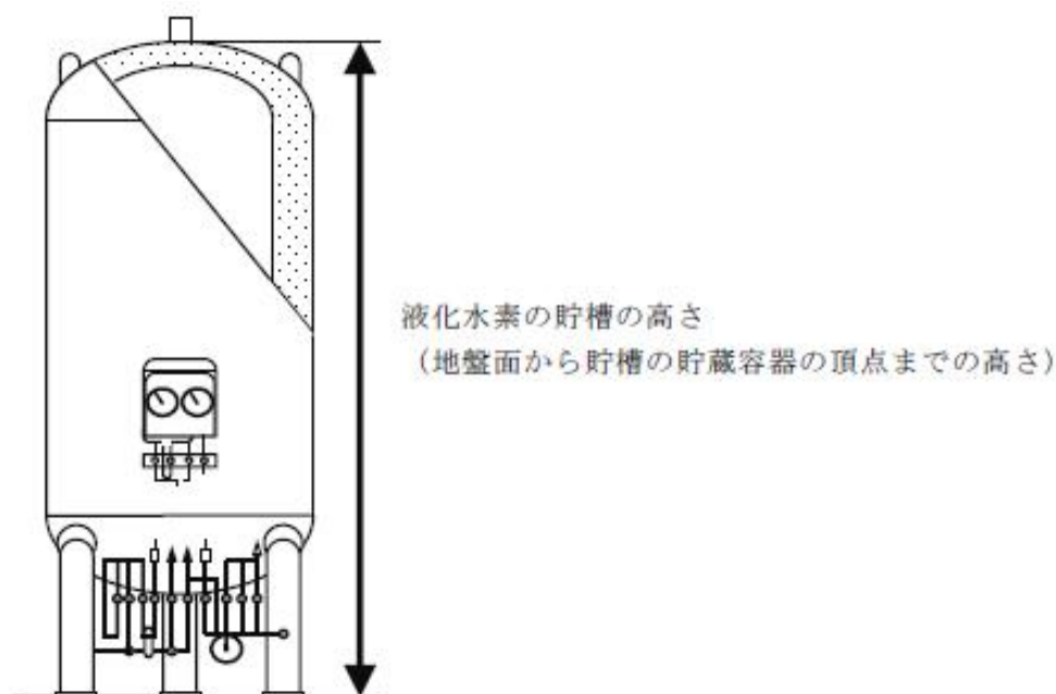
第12-61 図 液化水素の貯槽の高さ
