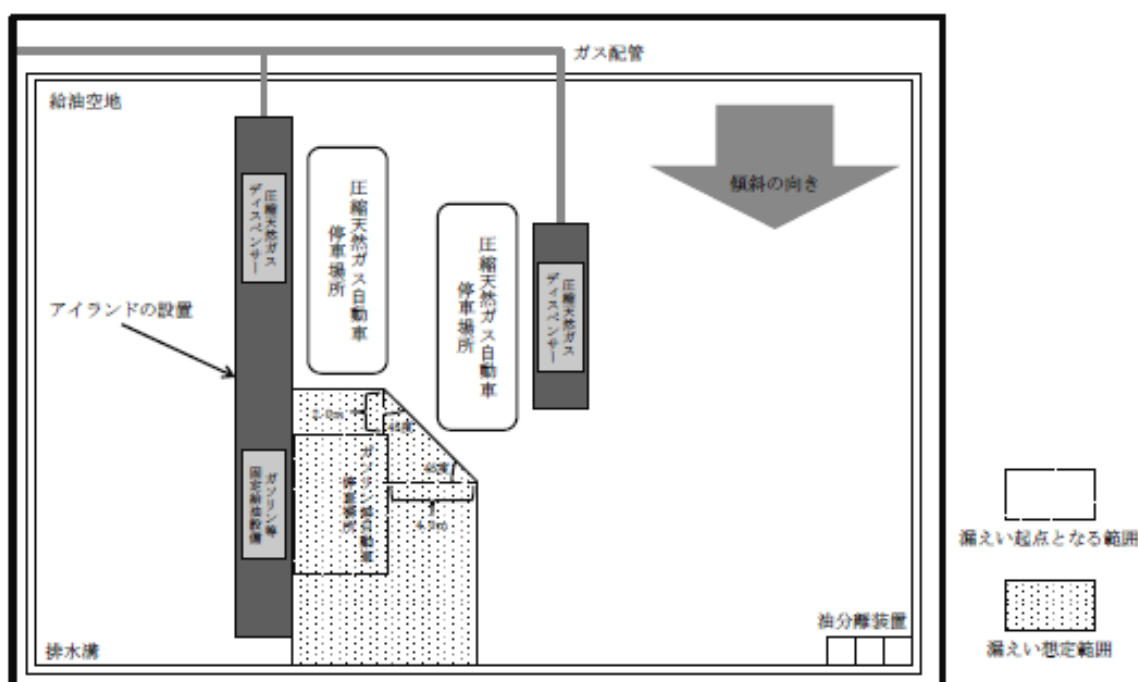
第 12- 59 図 圧縮天然ガススタンドのディスペンサー及びガス配管を給油空地に設置する例 1
