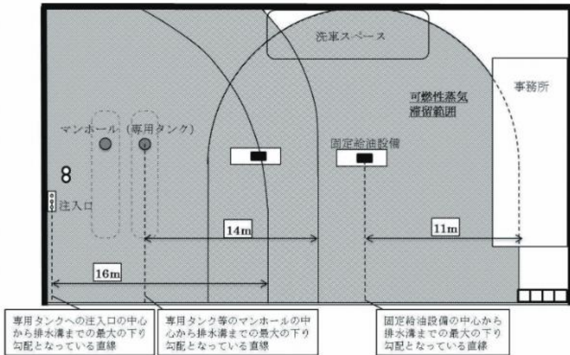
第 12-38 図 給油取扱所（平面図）で危険物の流出その他の事故により発生した可燃性の蒸気が滞留するおそれのない場所（斜線部分以外）
