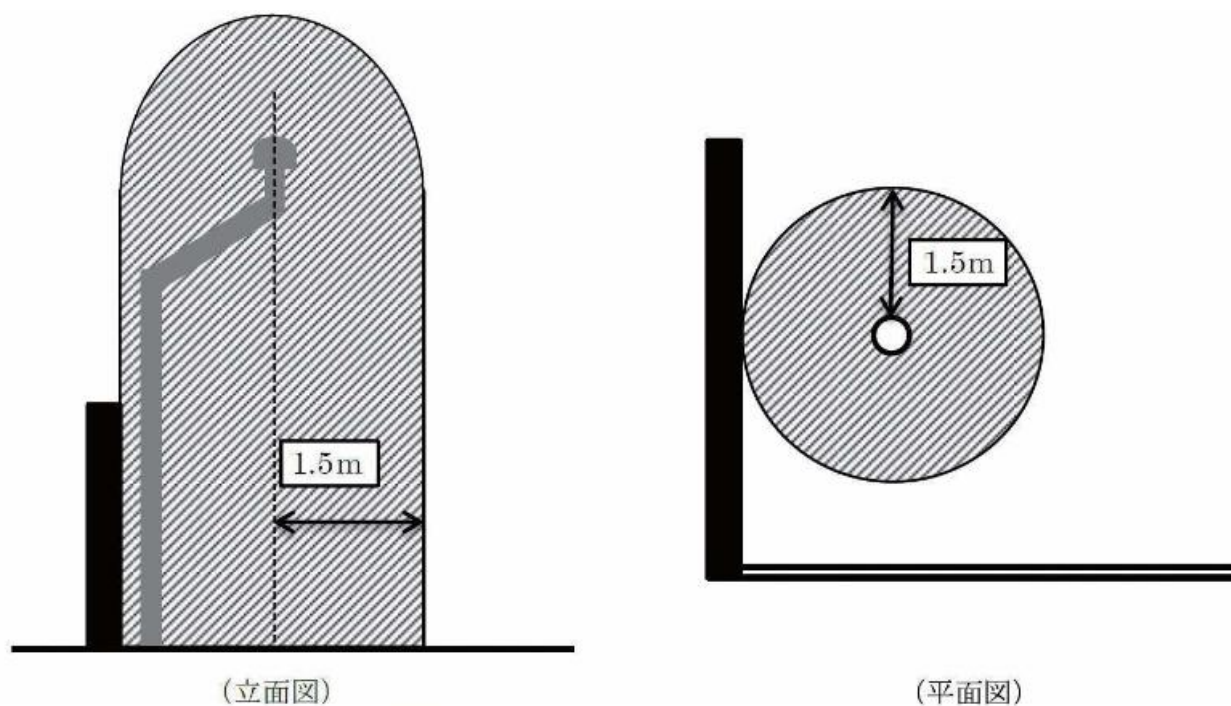
第 12-37 図 通気管の周囲で危険物の流出その他の事故により発生した可燃性の蒸気が滞留するおそれのない場所（斜線部分以外）
