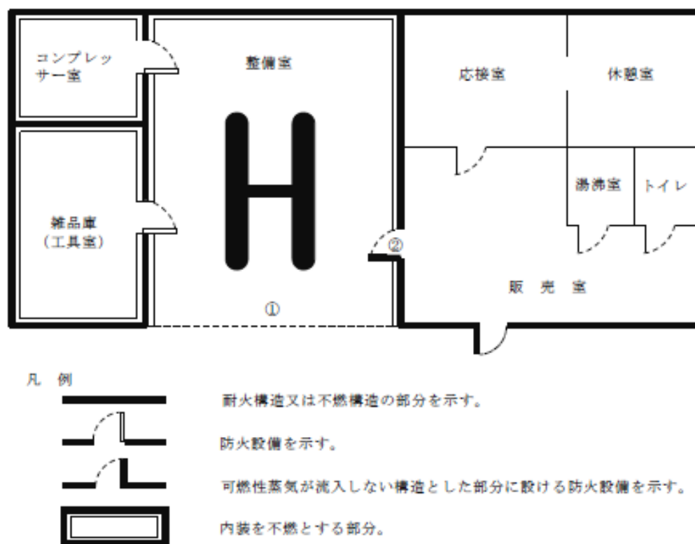
第12-18図 内部構造例
