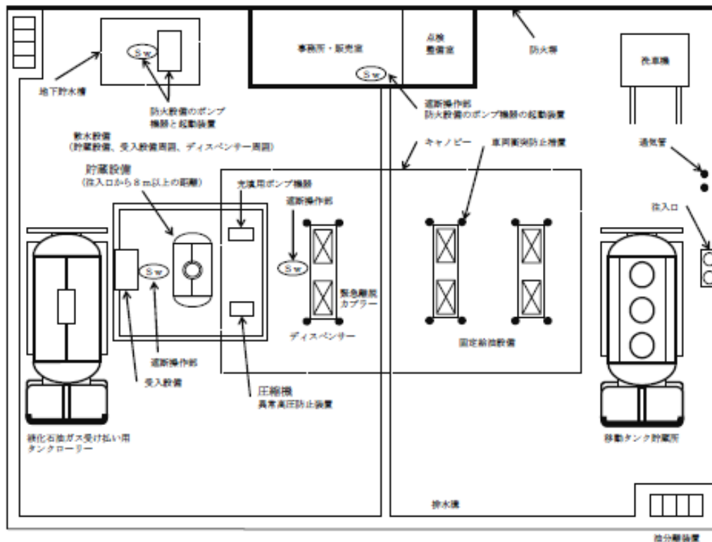
第 12- 55 図 屋外給油取扱所に液化石油ガススタンドを併設した例
