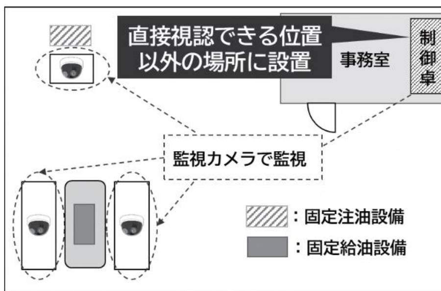
第 12-78 図 全ての顧客用固定給油設備等の使用状況を監視設備により視認できる位置に制御卓を設置する例
