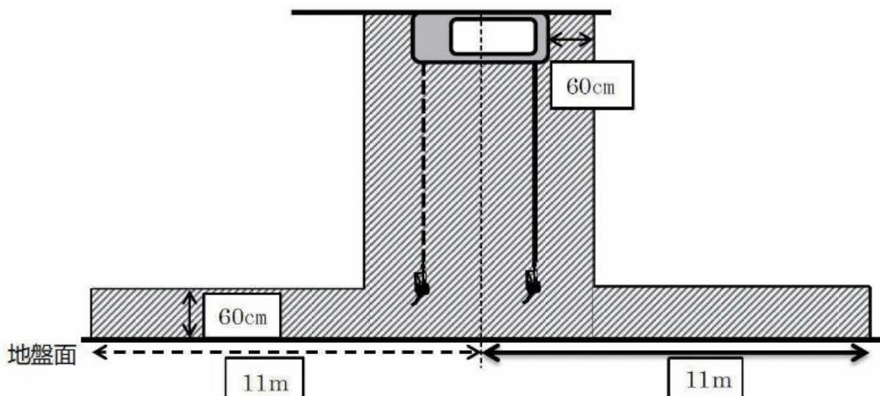
第 12-36 図 懸垂式の固定給油設備の周囲で危険物の流出その他の事故により発生した可燃性の蒸気が滞留するおそれのない場所（斜線部分以外）
