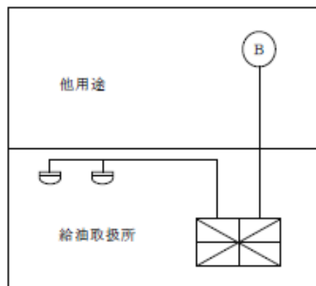
第 12- 45 図 他用途に報知する設備の例
