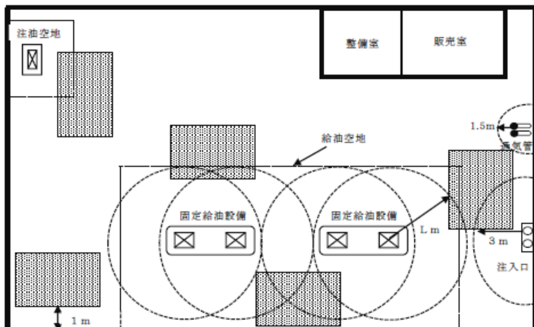
第12-15図 作業場等（網かけ部分）として認められない設置例
