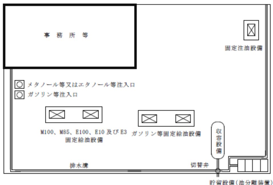
第 12- 66 図 給油空地等の周囲に排水溝等を設ける場合（注入口に係る排水溝と兼用）の例
