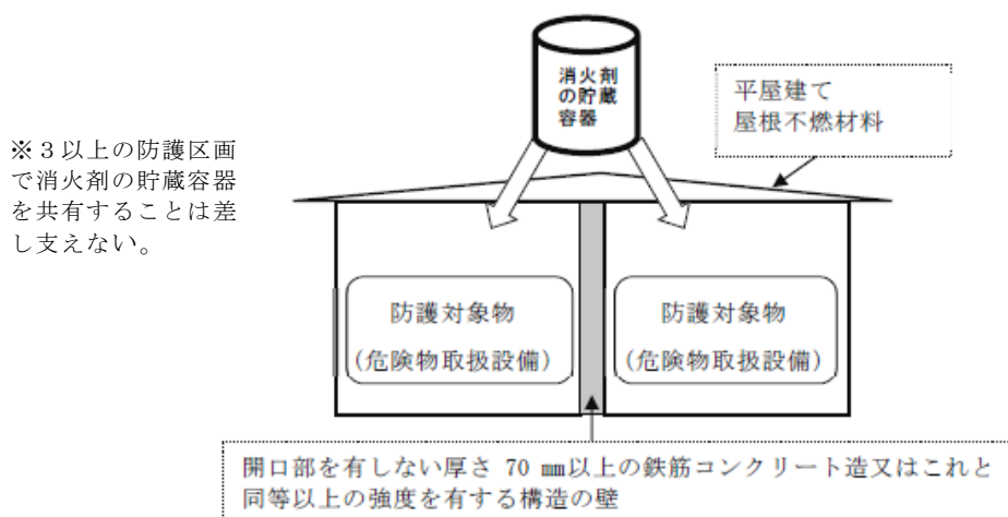
第17-9 図 防護対象物が互いに隣接する場合の消火剤貯蔵容器の共用例2
