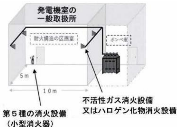
第17-2 図 区画室単位の一一般取扱所に特例基準を適用した場合の例
