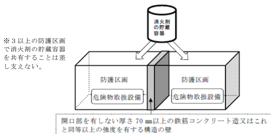
第17-8 図 防護区画が互いに隣接する場合の消火剤貯蔵容器の共用例1
