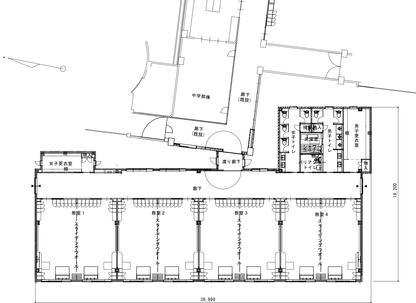
1 階平面図
