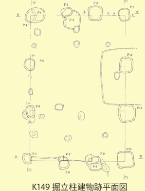
K149 掘立柱建物跡平面図
